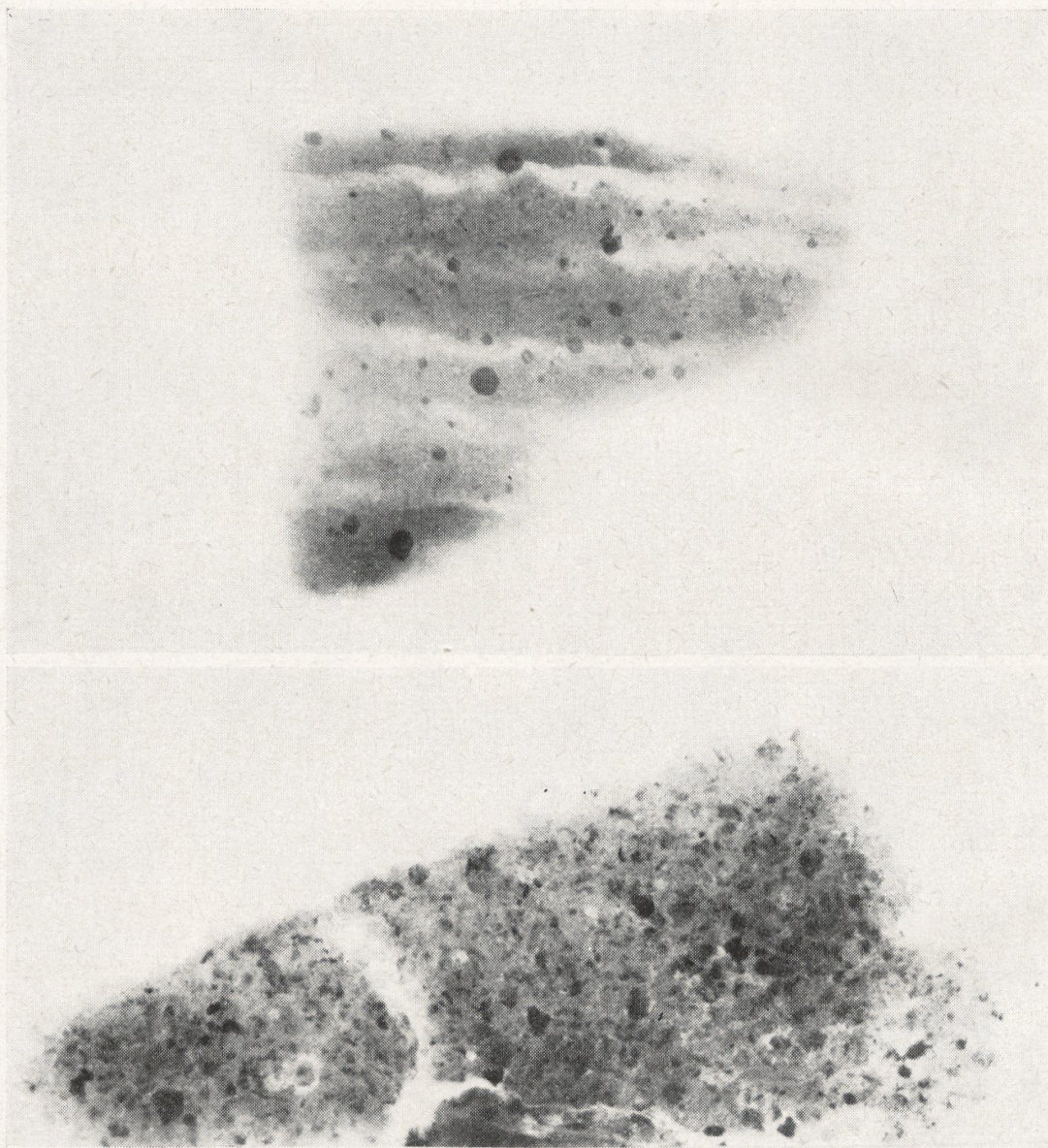
Röntgenaufnahmen zweier Tonscherben mit darinbefindlichen Eisenkonglomeraten in Kügelchenform, nat. Gr.
