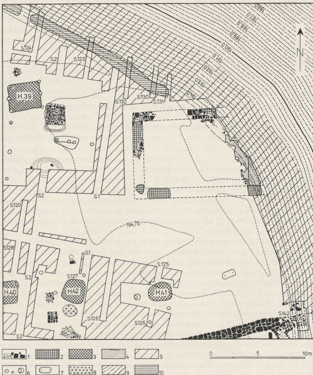
Abb. 3. Nordostecke der Hauptburg mit der Halle. Nach P. Grimm 1963 mit Verbesserungen. 1 Stein; 2 Kalkmörtel; 3 Hausverfärbung; 4 Gipsestrich; 5 nicht ausgegraben; 6 Pfosten oder flache Grube; 7 Mörtelpfanne; 8 zerstörte Öfen; 9 Höhenlinien; 10 Reste der nördlichen Umfassungsmauer
