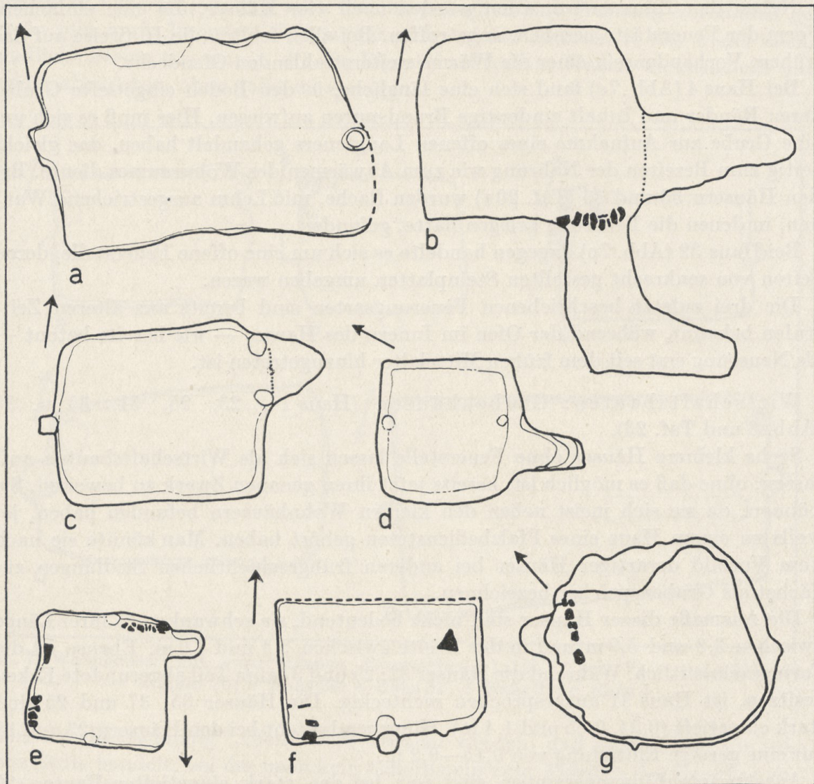
Abb. 8. Grubenhäuser und Eisenverarbeitungsstelle. 1:125. Nach P. Grimm 1960—64. a Haus 23; b Haus 25; c Haus 35; d Haus 37; e Haus 14; f Haus 31; g Haus 1
