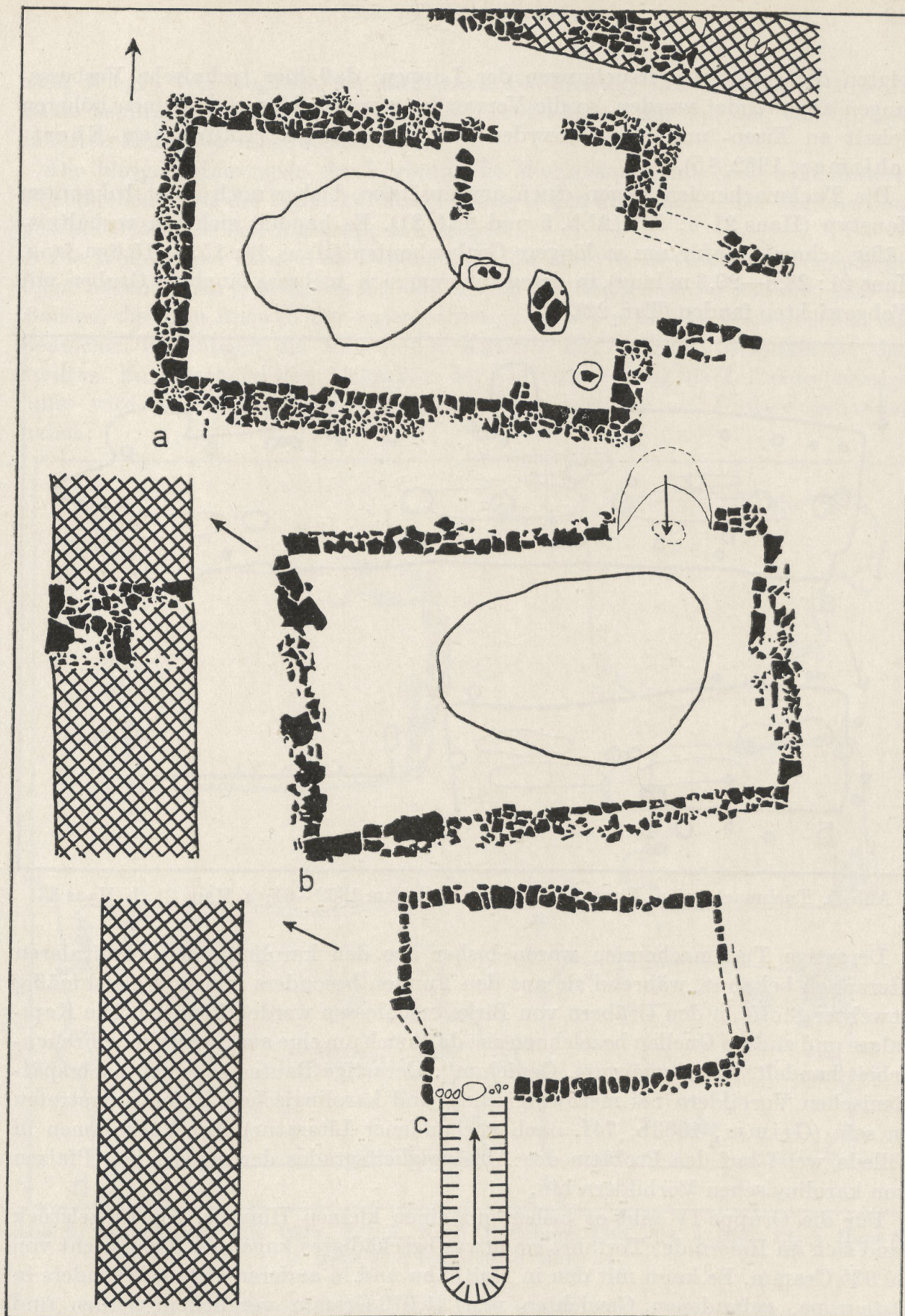
Abb. 4. Wachhäuser hinter der Umfassungsmauer der Vorburg. 1:125. Nach P. Grimm 1960–64; a Haus 11; b Haus 3; c Haus 2
