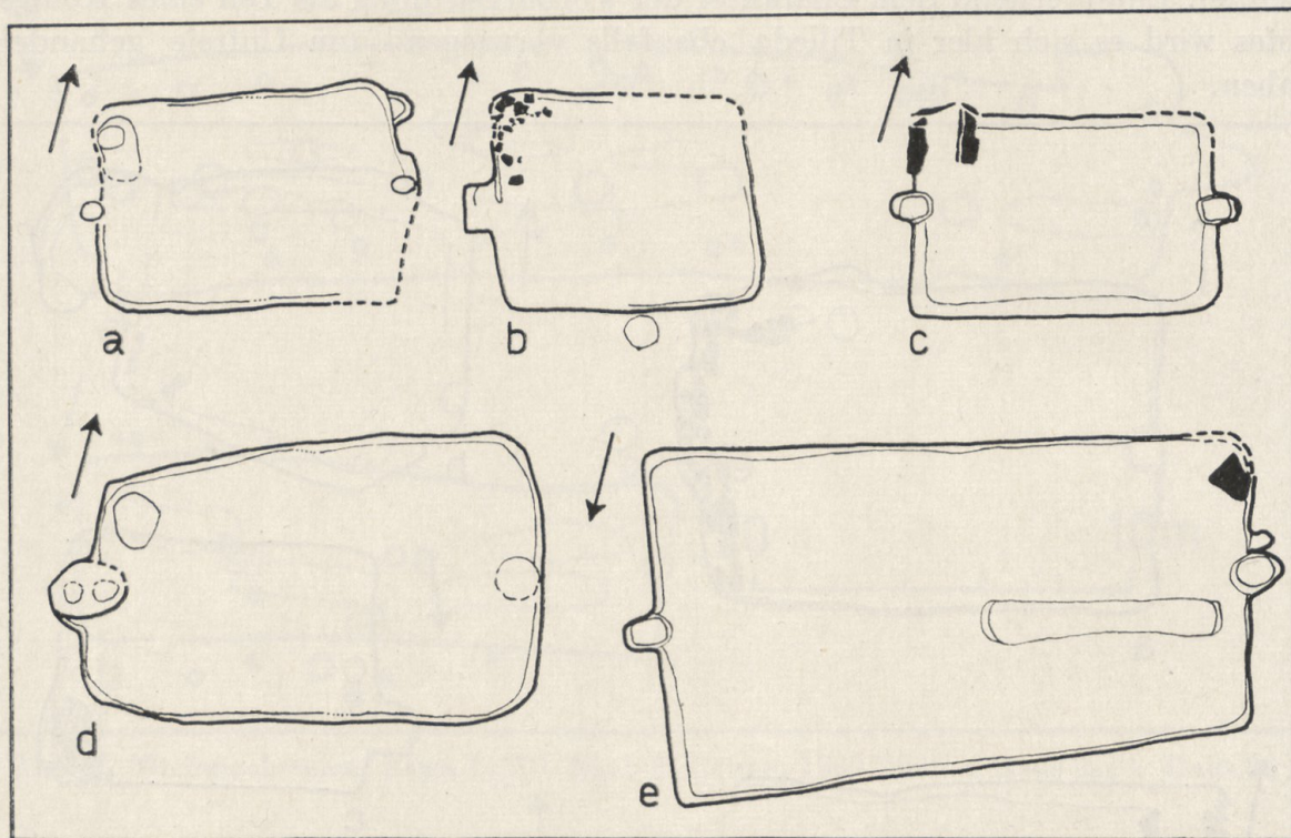
Abb. 7. Wohnhäuser mit verschiedenen Feuerstellen. 1:125. Nach P. Grimm 1961—64. a Haus 20; b Haus 34; c Haus 32; d Haus 36; e Haus 4
