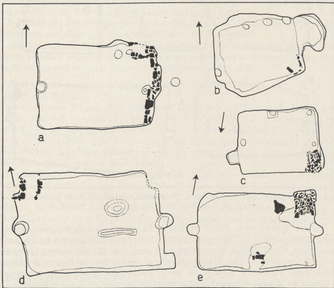
Abb. 6. Wohnhäuser mit Öfen. 1:125. Nach P. Grimm 1961–64. a Haus 29; b Haus 6; c Haus 5; d Haus 30; e Haus 24
