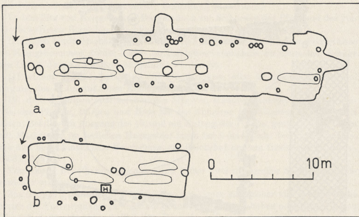
Abb. 5. Tuchmachereien. Etwa 1:275. Nach P. Grimm 1962—64; a Haus 21; b Haus 33
