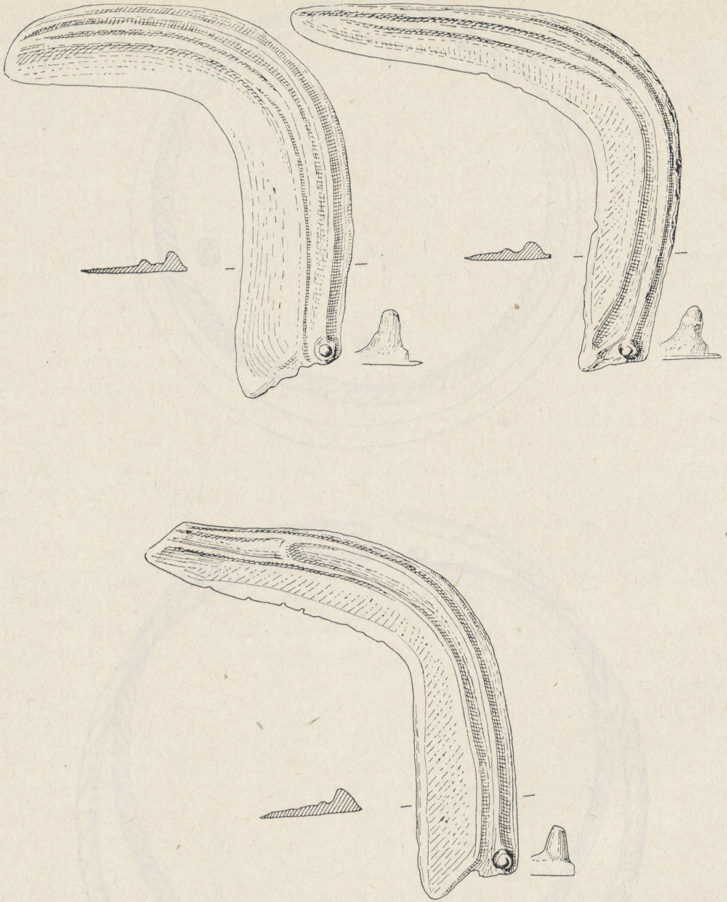
Abb. 21. Kloschwitz—Beesenstedt, Saalkreis. Hortfund, Sicheln (Fundteil Mus. Jena) (nach W. A. v. Brunn, 1954, b) 1:2
