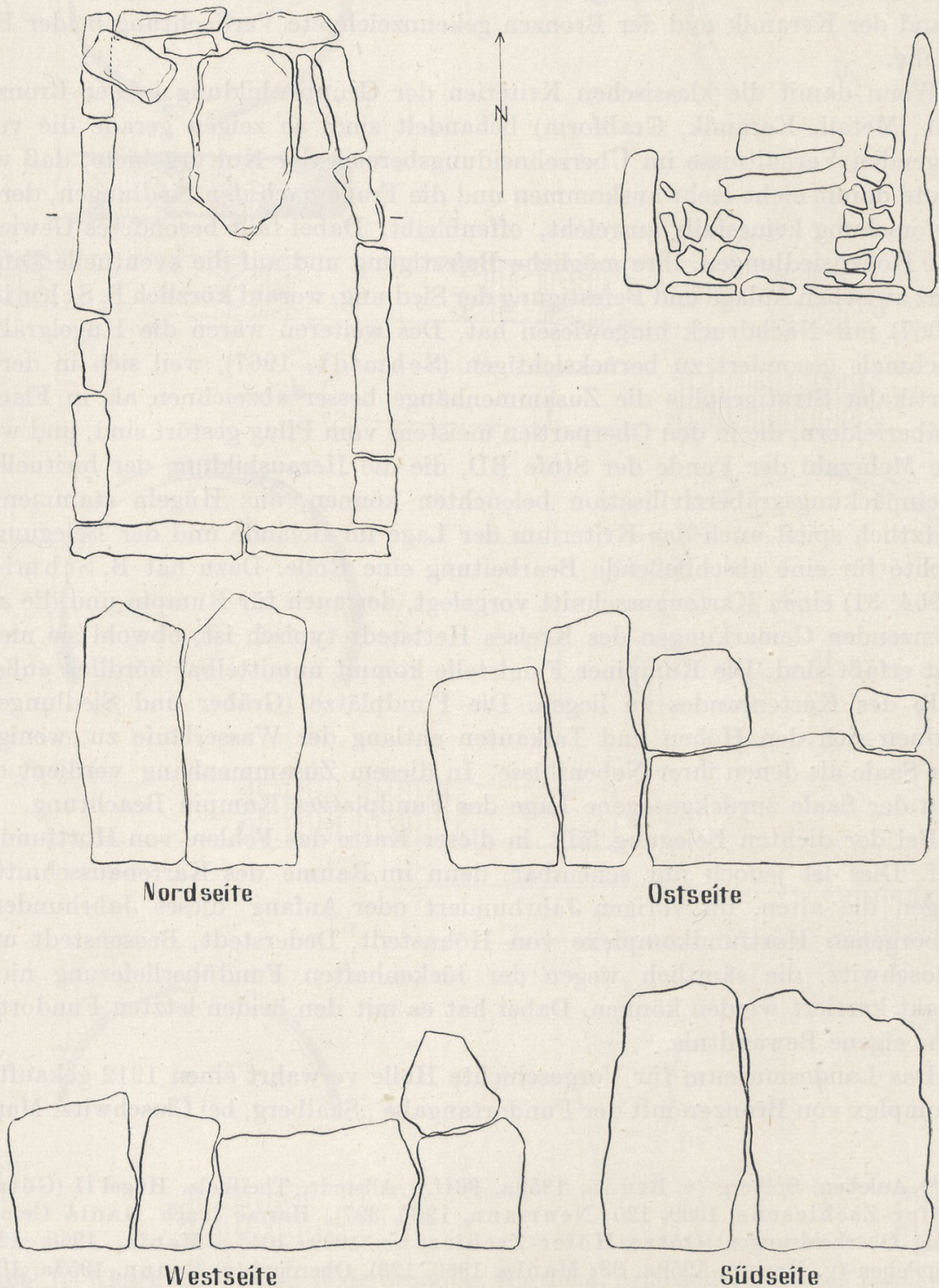
Abb. 12. Polleben, Kr. Eisleben. Grab, Steinkiste um Steinpackung (nach Fundbericht N. Niklasson, vgl. Anm. 34). 1:50
