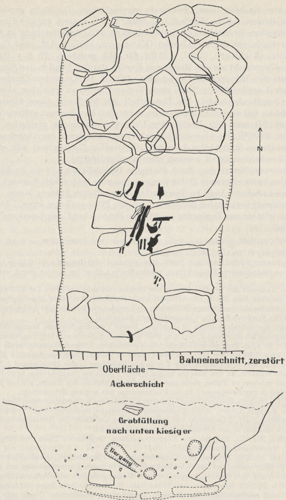
Abb. 10. Leuna, Kr. Merseburg. Grab, oben Steinpflaster, unten Schnitt (nach Fundbericht H. Hahne). 1:20
