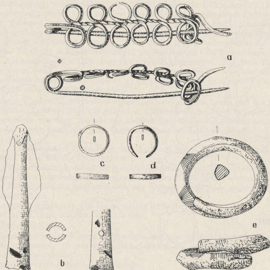
Abb. 9. Zabenstedt, Kr. Hettstedt. Grab 2, Bronzen. 1:2
