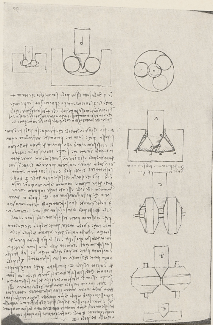
Abb. 1 Leonardo da Vinci: Rollen- und Kugellager. Madrid, Biblioteca Nacional, Cod. 8937, fol. 101v
