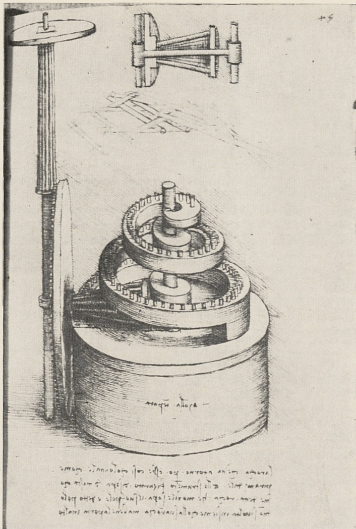
Abb. 2 Leonardo da Vinci: Getriebe mit gezahnter Spirale. Madrid, Biblioteca Nacional, Cod. 8937, fol. 45r
