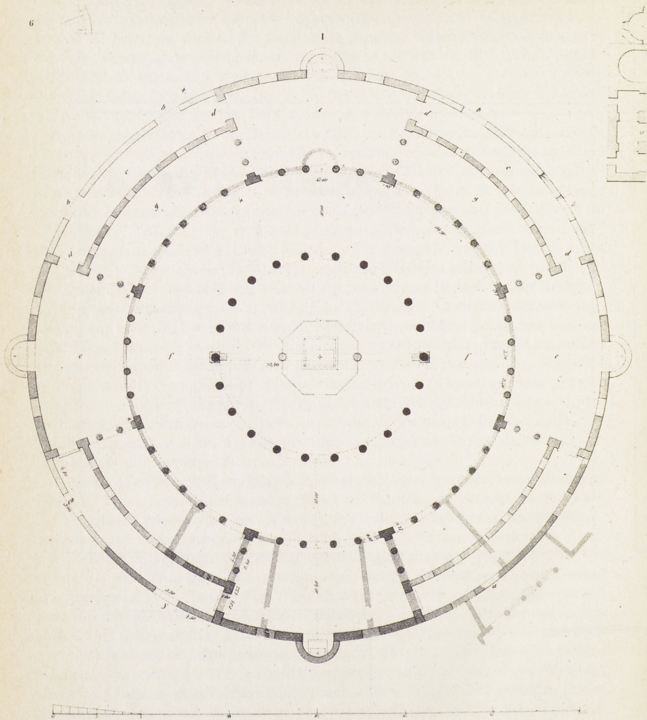
Fig. 3 H. Hübsch, Grundriß von S. Stefano Rotondo
