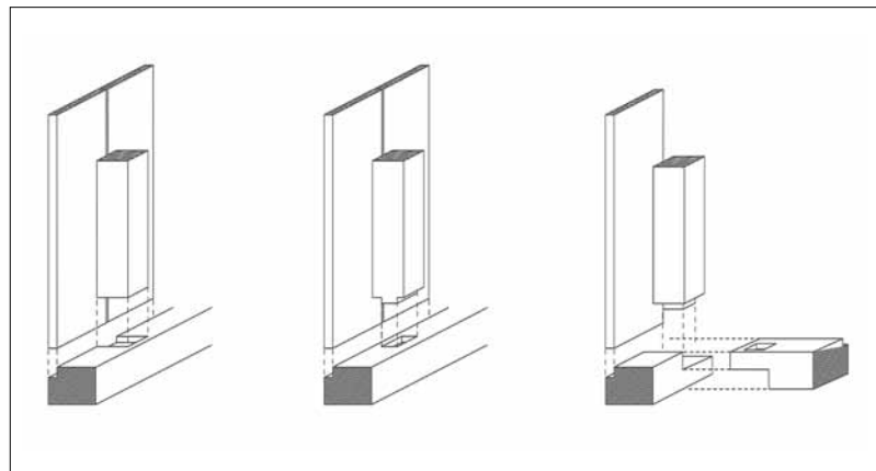
Abb. 12: Konstruktionsschemata der Zapfen- und Verblättungsverbindungen zwischen den Schwellen und den Ständern des unter- kellerten Schwellenständerbaus an der Braun- straße 30A/B.
