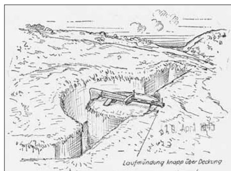
Abb. 5: Schema eines MG-Stands aus dem Handbuch „Der kleine Stellungsbauer“.
