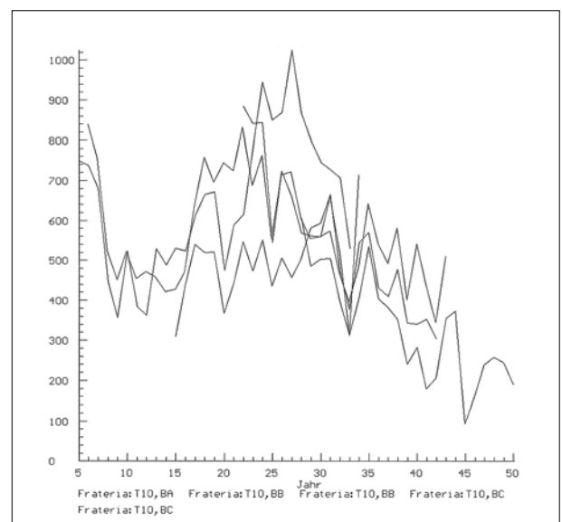
Abb. 20: Frateriatür, datierte Radien der Bohlen A–C in ihrem zeitlichen Verhältnis zueinander.
