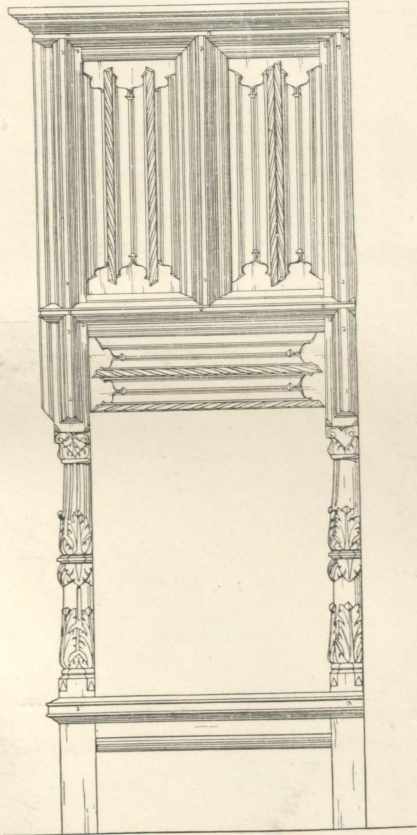
Seitenansicht.
