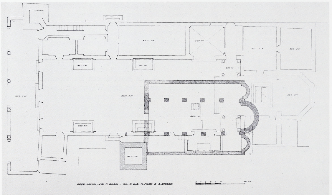
14 Impruneta, Sanktuarium S. Maria dell'Impruneta. Grundriss mit Eintragung der verschiedenen Bauperioden. Zeichnung: Fossi/Bigazzi.
