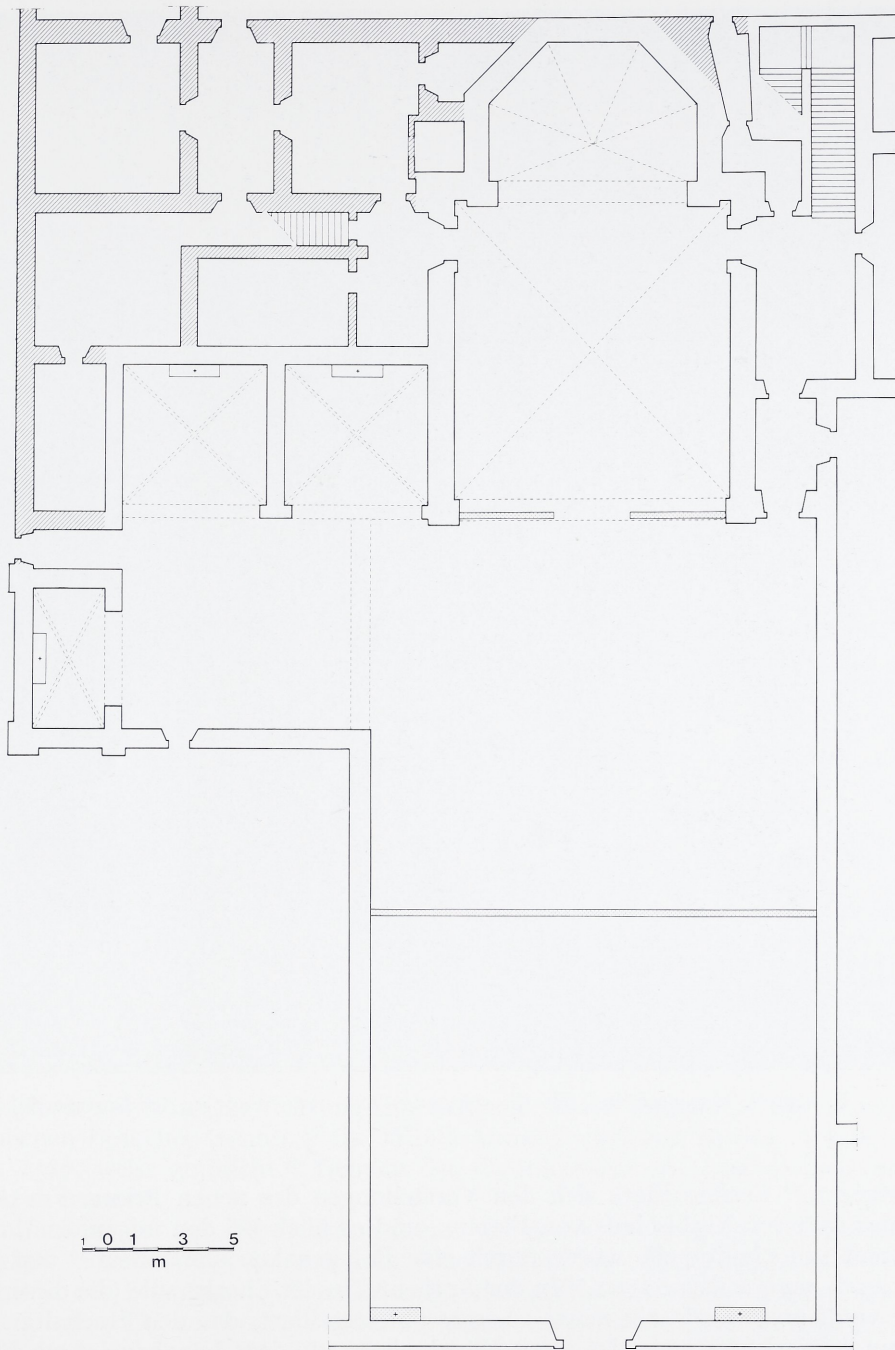
8 Florenz, S. Marco. Grundriss, schematische Rekonstruktion der Kirche nach dem Umbau von 1438 ff. (schraffiert: nach 1500 angefügte Bauteile; punktiert: hypothetische Details). Zeichnung: M. Ferrara nach Angaben des Verfassers.
