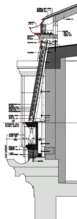
1 Karlsruhe, Erbgroßherzogliches Palais, Planschnitte durch die Konstruktion zur Erneuerung der Mansarde.
