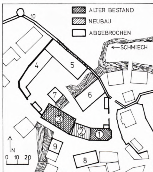
1 EHINGEN, HEILIG-GEIST-SPITAL. Der Lageplan zeigt die ursprüngliche Anlage und den heutigen Bestand. 1 = Kirche, 2 = Amtshaus, 3 = Neuhaus, 4 = Roßstall, 5 = Großer Stadel, 6 = Neuer Stadel, 7 = Neues Häusle, 8 = Stadel, 9 = Mühle, 10 = Stadtmauer.
