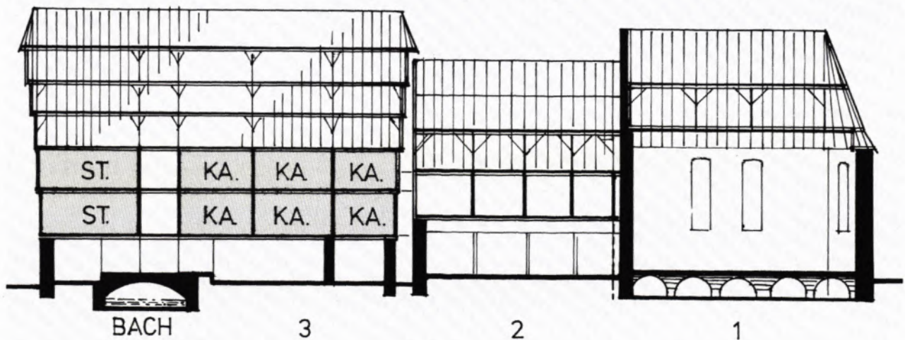
3 LÄNGSSCHNITT DURCH NEUHAUS, AMTSHAUS UND KIRCHE. Der Querflur zwischen Stube und Kammern im Neuhaus liegt genau über dem Bachlauf. Der Winkel zwischen Neuhaus und Amtshaus wurde später baulich geschlossen.
