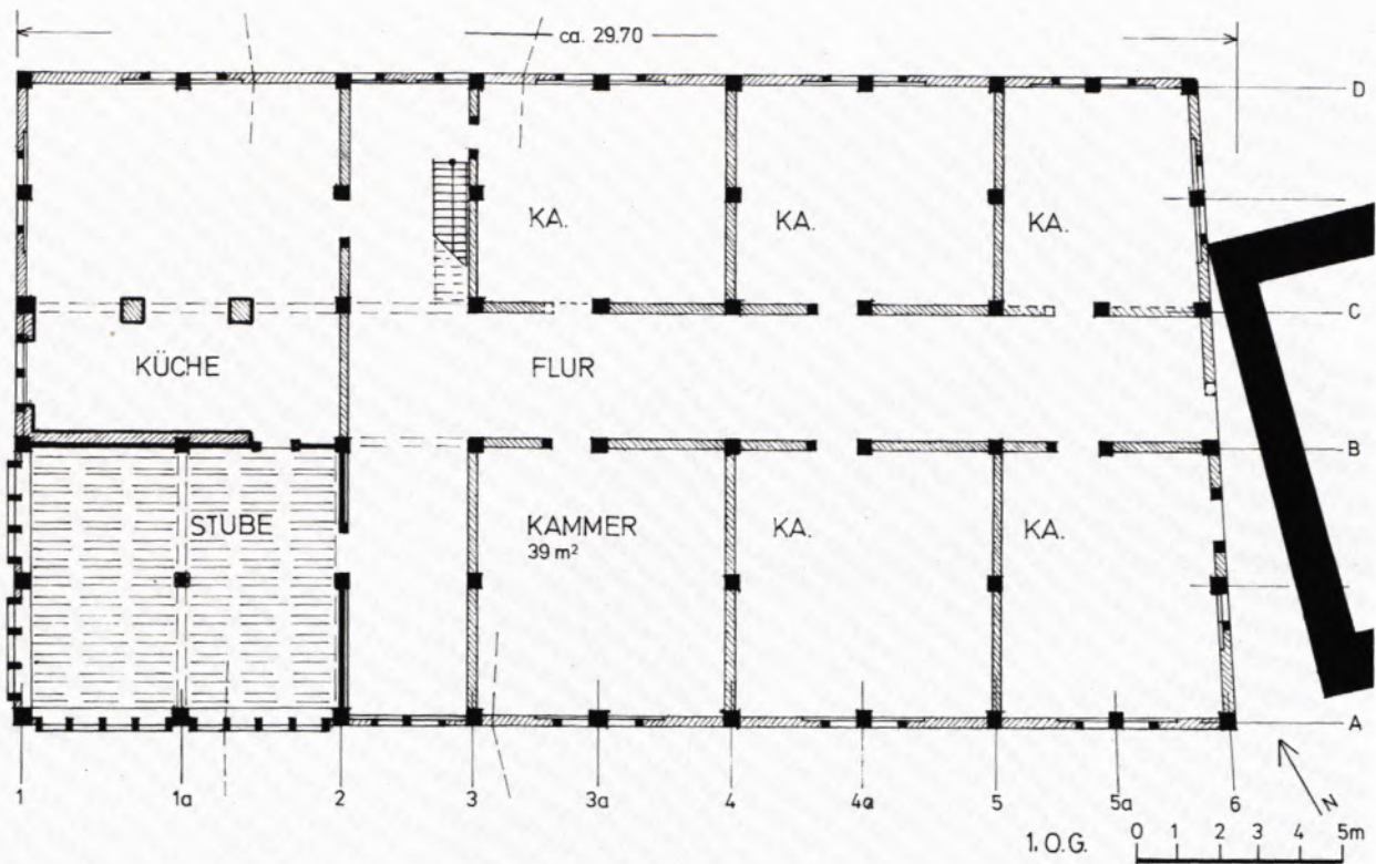
2 EHINGEN, NEUHAUS des Heilig-Geist-Spitals. Grundriß des ersten Obergeschosses. Mit Rücksicht auf das bestehende Amtshaus (rechts) wurde der anschließende Giebel des Neuhauses schräg geführt. Offenbar waren der vordere Giebel und die Länge des Hauses mit 100 Fuß genau festgelegt.
