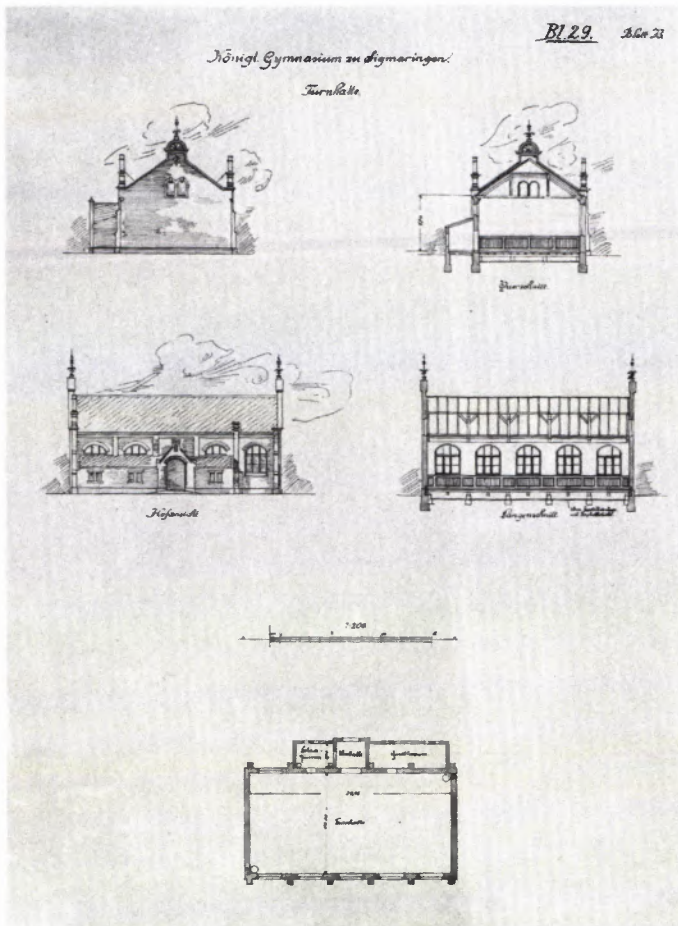
9 AUSFÜHRUNGSENTWURF DER TURNHALLE IN SIGMARINGEN VON 1891.
