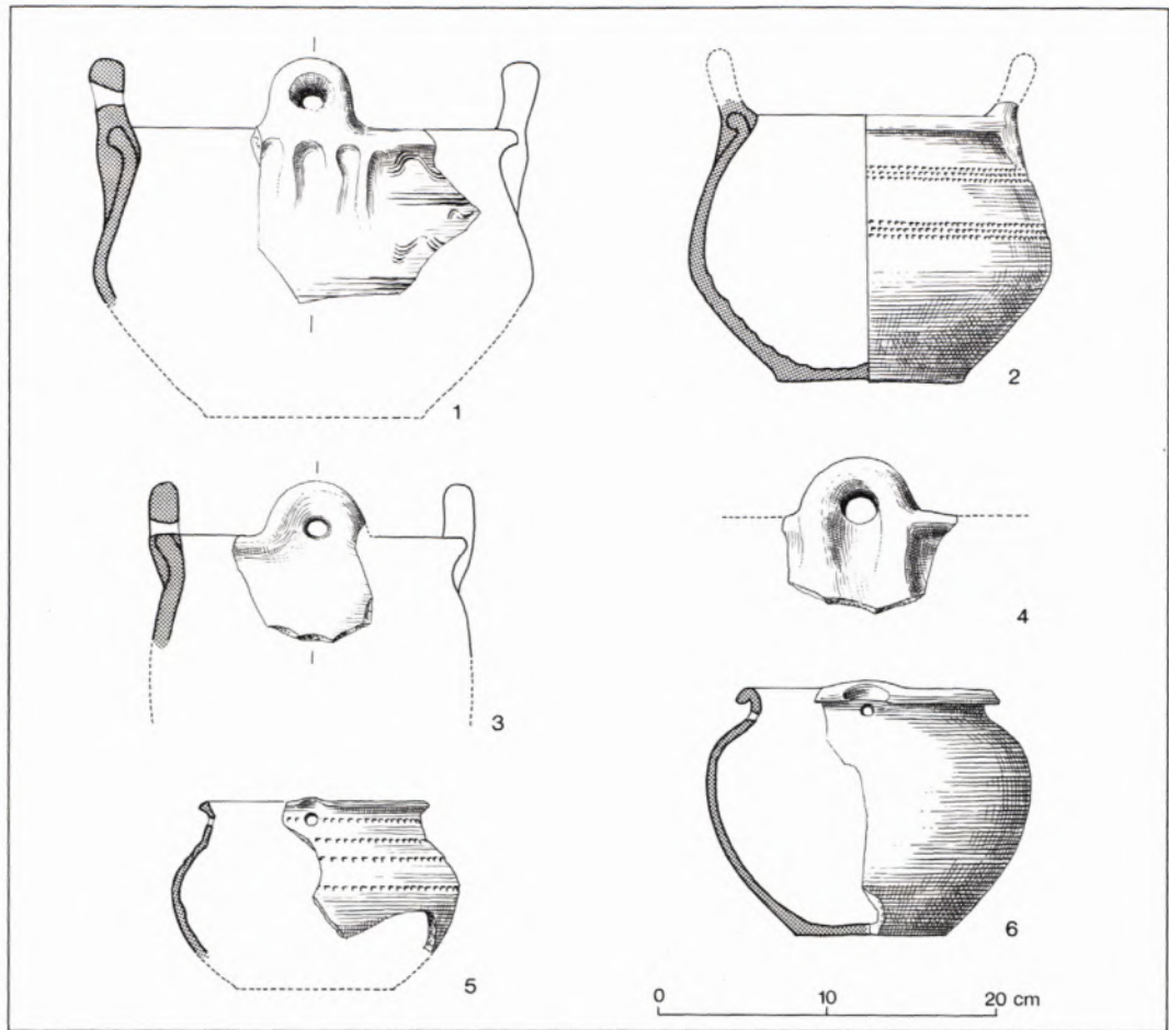
5 HÄNGE- GEFÄSSE aus Mannheim-Vogel- stang (1), Ried- stadt-Crumstadt (2), Wülfingen (3), Königsbronn (4), Ensisheim, dép. Haut-Rhin (5), Hohenfels/Eifel (6). M. 1:4.
