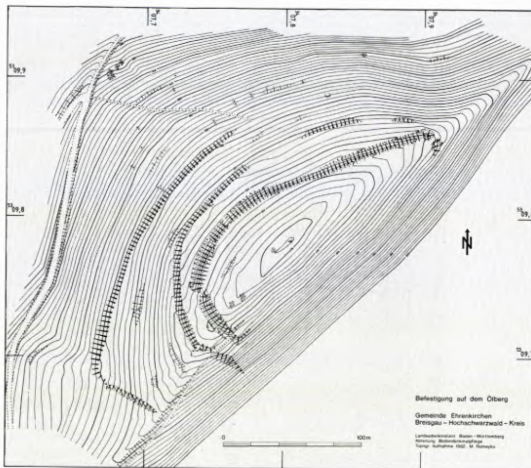
11 VORGE-SCHICHTLI-CHE Befestigungsanlage auf dem Ölberg bei Ehrenstetten, Kr. Breisgau-Hochschwarzwald. Aufgenommen für das LDA durch M. Romejko 1982.
