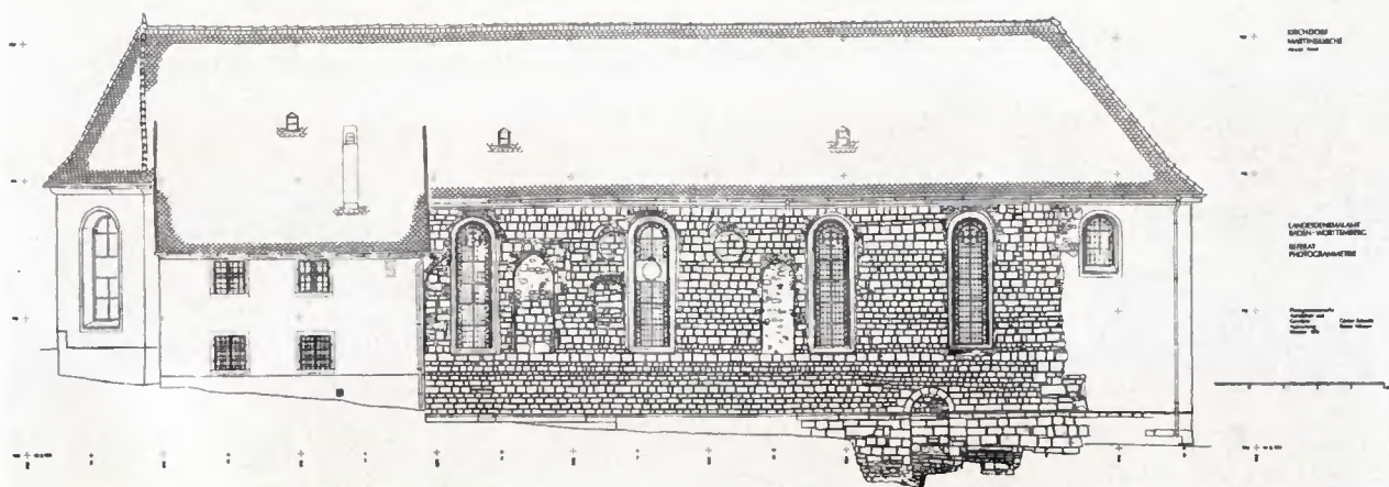
8 KIRCHDORF, Schwarzwald-Baar-Kreis. Nordansicht der Martinskirche mit bauarchäologischen Befunden verschiedener Perioden, aufgenommen bei Beginn der Renovierungsarbeiten 1978.
