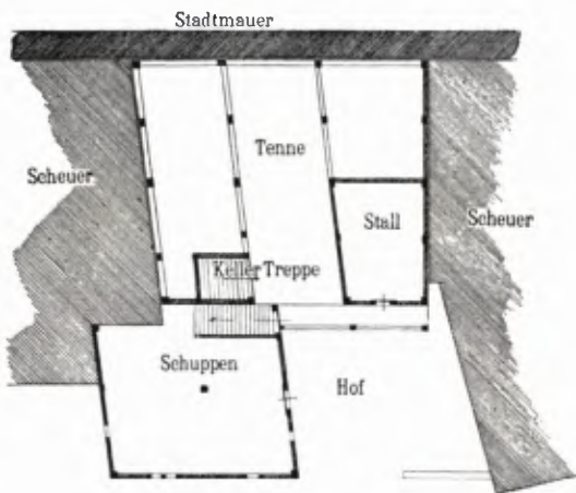
Abb. 9b. Erdgeschoß.
