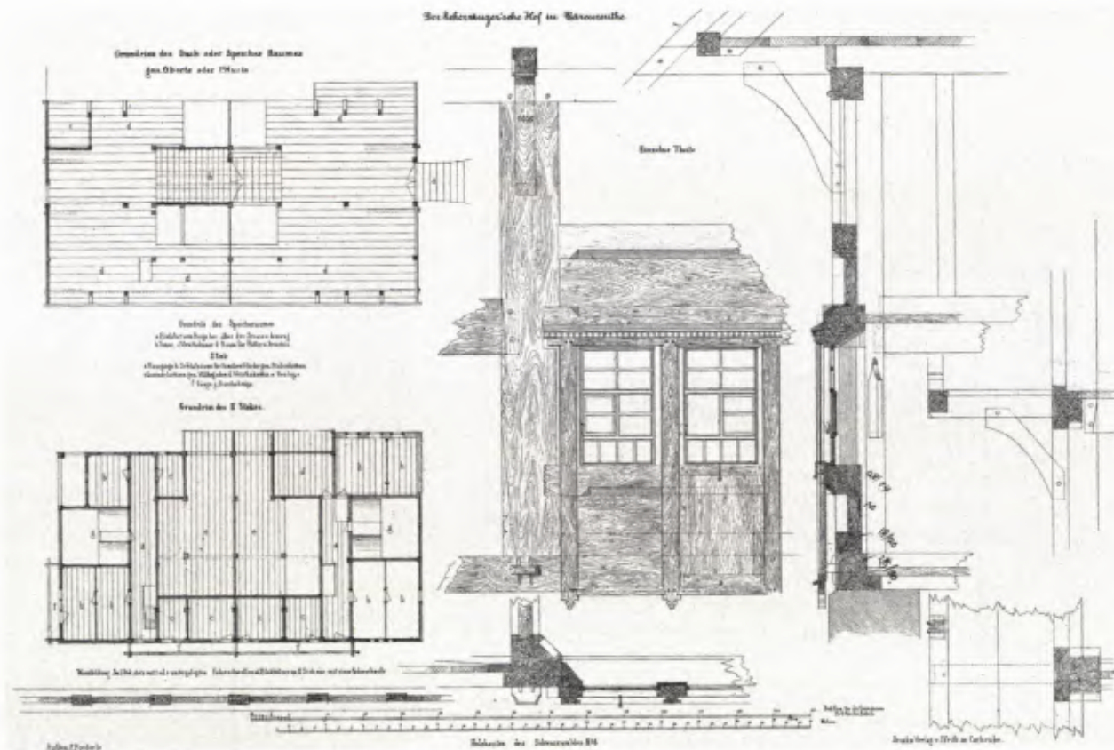
3 SCHÄRZINGERSCHER HOF BÄRENREUTHE, Gde. Bregenbach (heute Stadt Vöhrenbach, Schwarzwald-Baar-Kreis), aus: „Holzbauten des Schwarzwaldes“ von Friedrich Eisenlohr, aufgenommen von F. Feederle 1853. Das Werk markiert den Beginn der wissenschaftlichen Bauernhausforschung.
