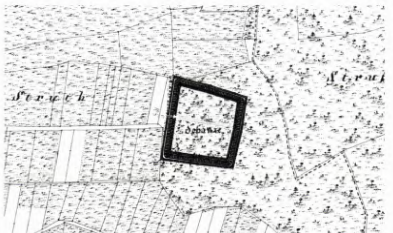
6 KELTSICHE Viereckschanze bei Langenburg, Kr. Schwäbisch Hall. M. 1: 5000. Aufgenommen von Major Steiner 1899.
