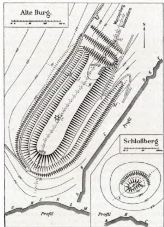
8 „ALT-HAYINGEN“ bei Hayingen-Indelhausen, Kr. Reutlingen. Verkleinerung des dreifarbigigen Originals in den Maßstab 1:5000. Aufgenommen von G. Kottmayer 1950.
