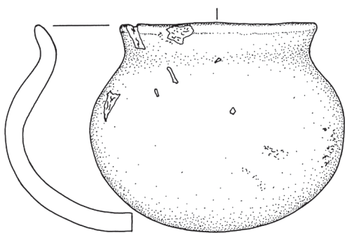
Abb. 15 Westeraccum OL-Nr. 2310/6:25, Gde. Dornum, Ldkr. Aurich (Kat.Nr. 14) Frühmittelalterlicher kleiner Kugeltopf. M. 1:2. (Zeichnung: S. Starke)
