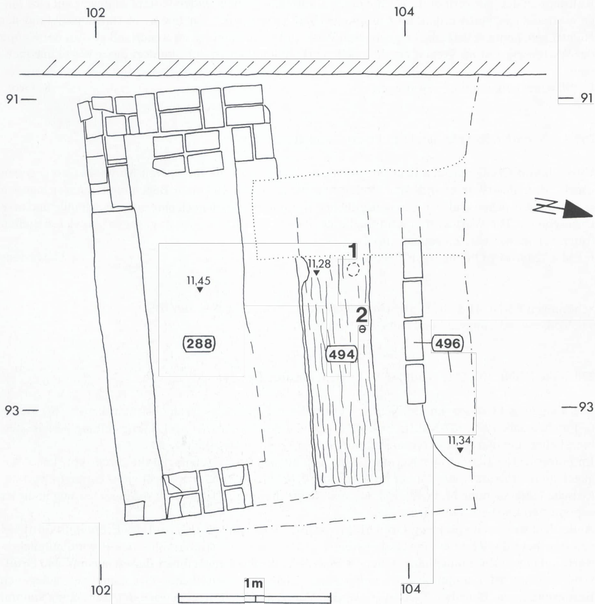
Abb. 116 Stade FStNr. 161, Gde. Stadt Stade, Ldkr. Stade (Kat.Nr. 270) Prämonstratenserkirche St. Georg, Chorbereich des 14. Jh.s. Zwischen der Gruft 288 des Erzbischofs Gottfried von Arnsberg (Bestattung bereits entfernt) und dem Gruftrest 496 das Grab 494 mit „Beigaben“ (Skelett weitgehend vergangen und mit dem Sarg verbacken). 1 Lage des Blei-Zinn(?)-Bleches, 2 Gürtelschnalle.
