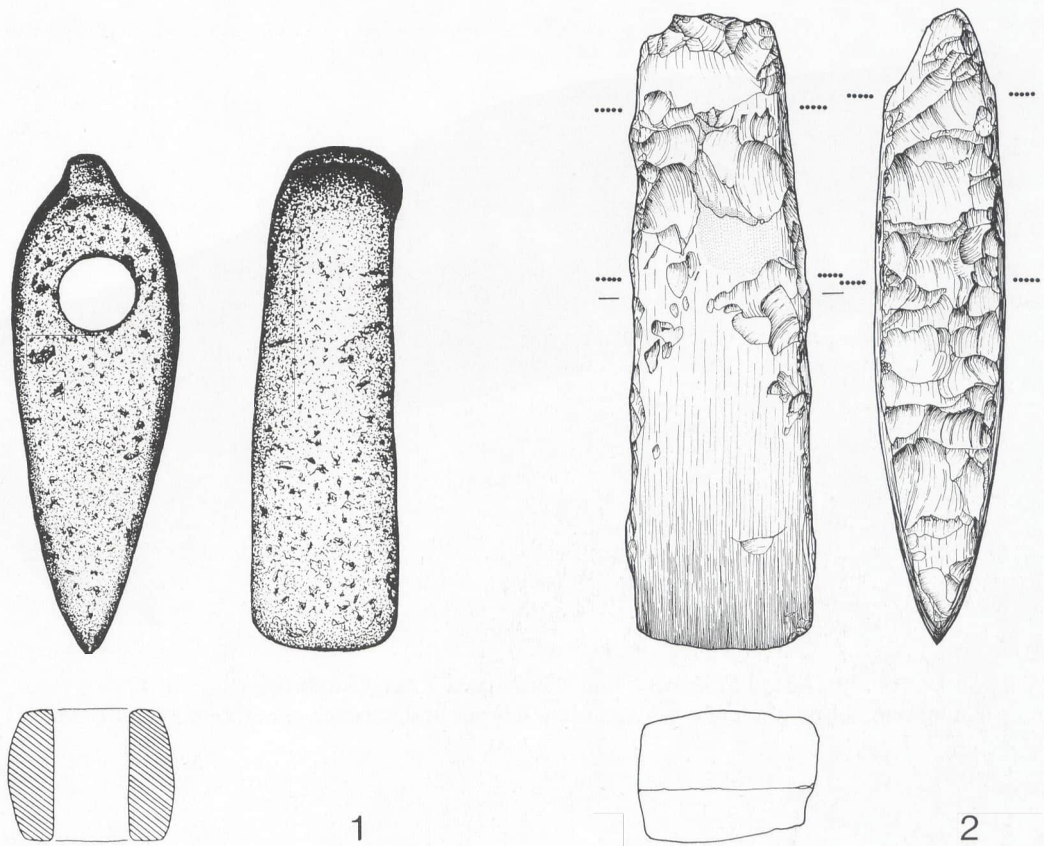
Abb. 29 1 Fallingbostel FStNr. oF 1, Gde. Stadt Fallingbostel, Ldkr. Soltau-Fallingbostel (Kat.Nr. 47) Streitaxt mit zusammengekniffenem Nacken. M. 1:2. 2 Flettmar FStNr. 1, Gde. Müden (Aller), Ldkr. Gifhorn (Kat.Nr. 48) Stumpfnackiges Flintrechteckbeil. Durch die gepunkteten Linien wird der Bereich der Schäftungspolitur angegeben. M. 1:2.
