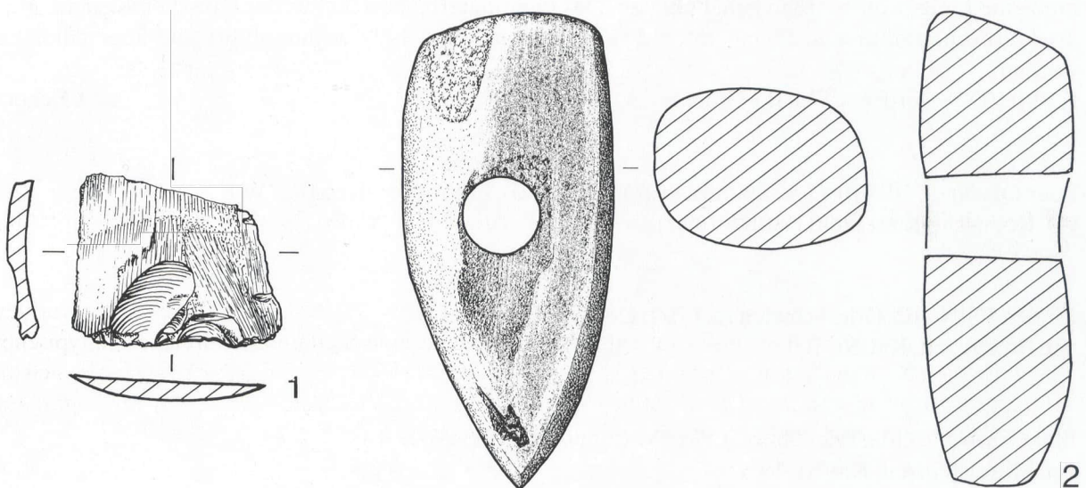
Abb. 35 1 Ippensen FStNr. 25, Gde. Vörden, Ldkr. Rotenburg (Wümme) (Kat.Nr. 62) Flintfragment; Absplitterung wohl von einem dickblattigen Beil der Einzelgrabkultur. M. 1:2. 2 Klein Vahlberg FStNr. 3, Gde. Vahlberg, Ldkr. Wolfenbüttel (Kat.Nr. 63) Durchbohrte Arbeitsaxt. M. 1:2.
