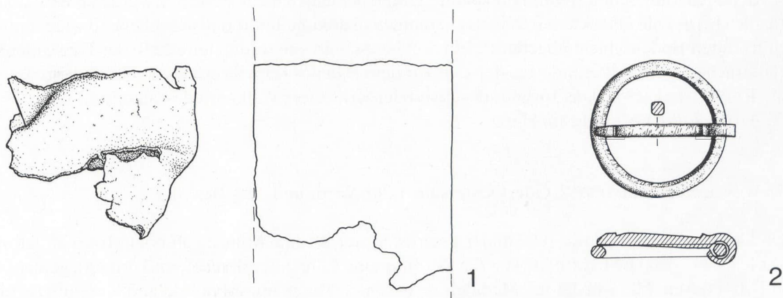
Abb. 117 Stade FStNr. 161, Gde. Stadt Stade, Ldkr. Stade (Kat.Nr. 270) Funde aus Grab 494: 1 Fragment eines Blei-Zinn(?)-Blechtes, 2 bronzene Gürtelschnalle. M. 1:2.
