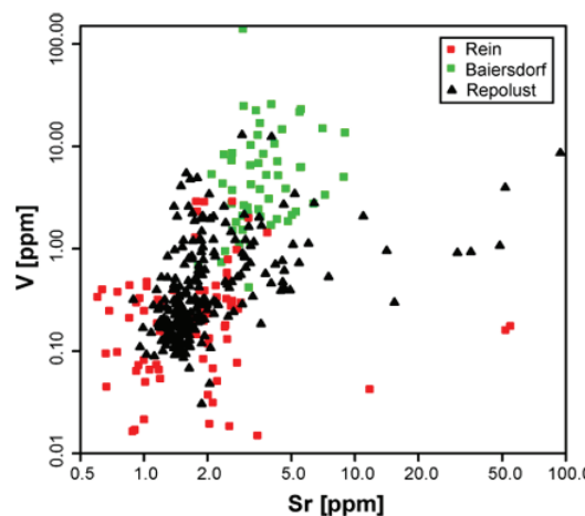
Fig. 16. Sr - V plot of Rein and Baiersdorf chert samples together with samples from the Repolust Cave. Abb. 16. Sr - V Plot von Reiner und Baiersdorfer Hornsteinproben zusammen mit Proben der Repolusthöhle.
