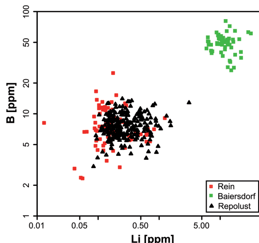
Fig. 14. Li - B plot of Rein and Baiersdorf chert samples together with samples from the Repolust Cave. Abb. 14. Li - B Plot von Rein und Baiersdorfer Hornsteinproben zusammen mit Proben der Repolusthöhle.
