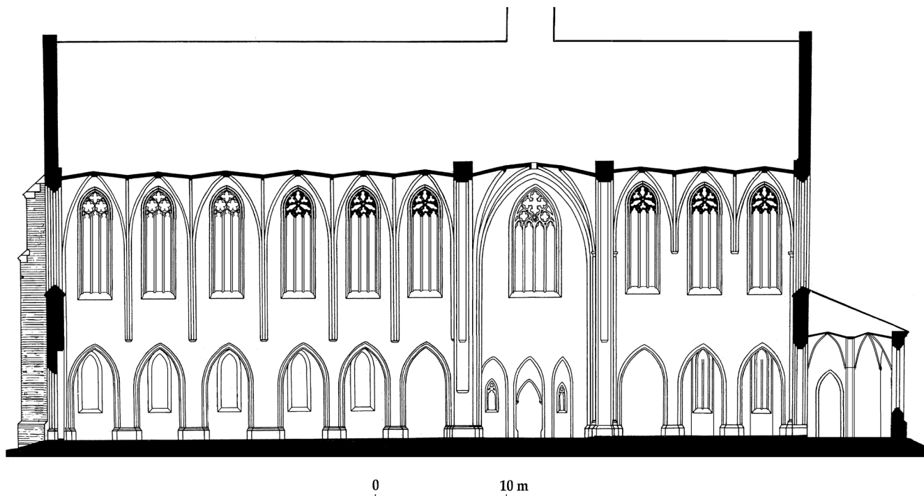
1. Lubiąż, kościół Cystersów, przekrój podłużny (rekonstrukcja pierwotnego wyglądu). Rys. J. Adamski Lubiąż, Cistercian Church, longitudinal section (reconstruction of the original appearance). Drawing: J. Adamski
