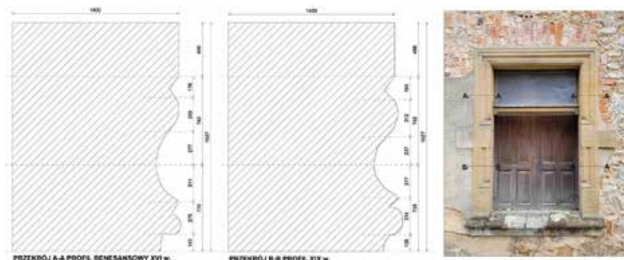
Ryc. 6. Wojcieszów, pałac, przekroje przez kamienne obramienia okienne, oprac. A Walkowska
