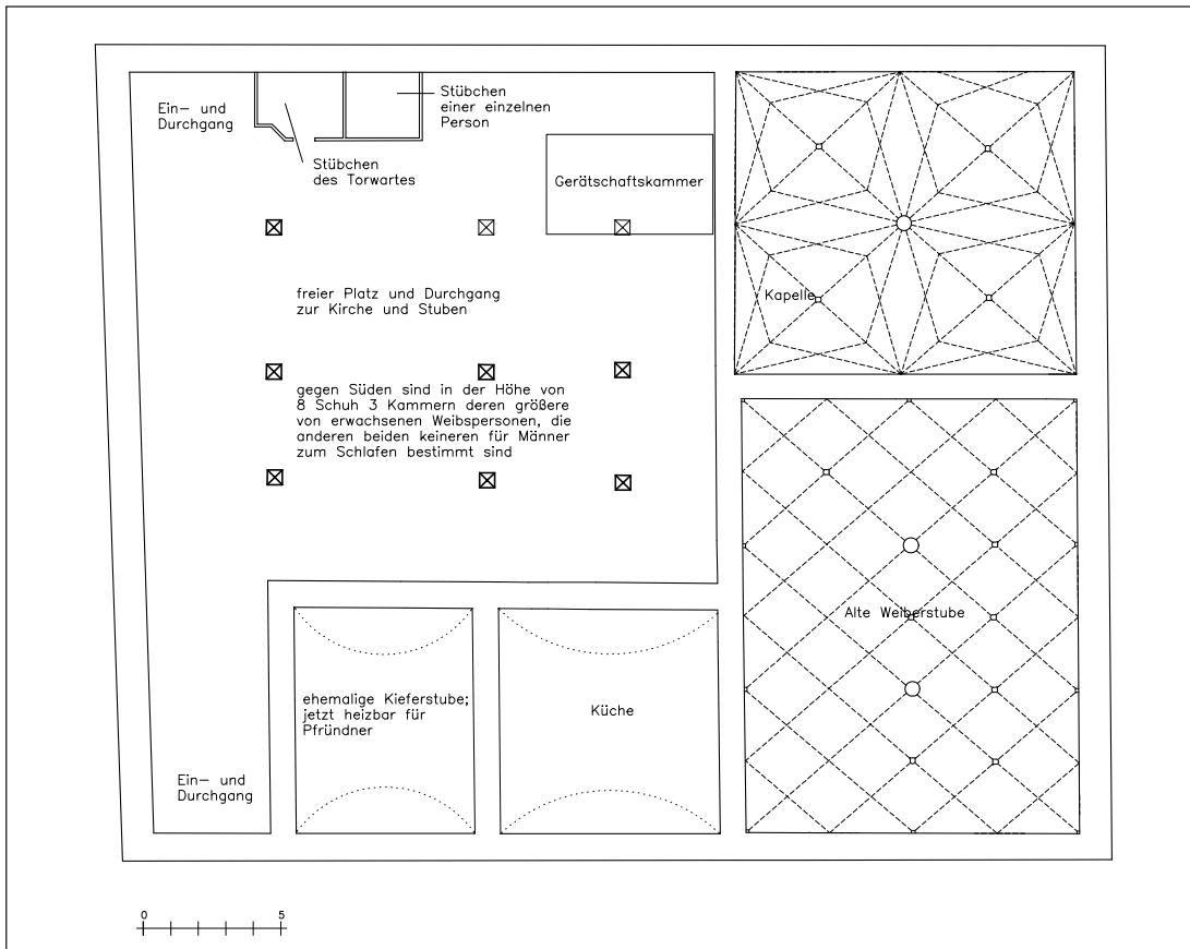
Abb. 7: Ravensburg, Heilig-Geist-Spital. Rekonstruktion um 1800, Erdgeschoss.
