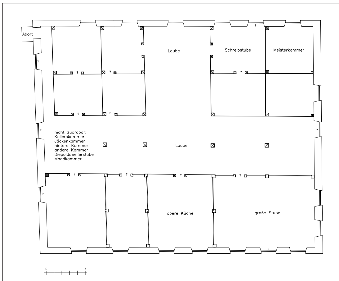
Abb. 3: Ravensburg, Heilig-Geist-Spital. Rekonstruktion um 1500, Obergeschoss.
