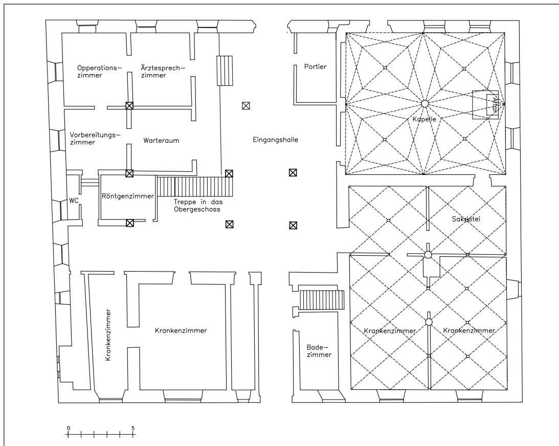
Abb. 10: Ravensburg, Heilig-Geist-Spital. Rekonstruktion um 1910, Erdgeschoss.
