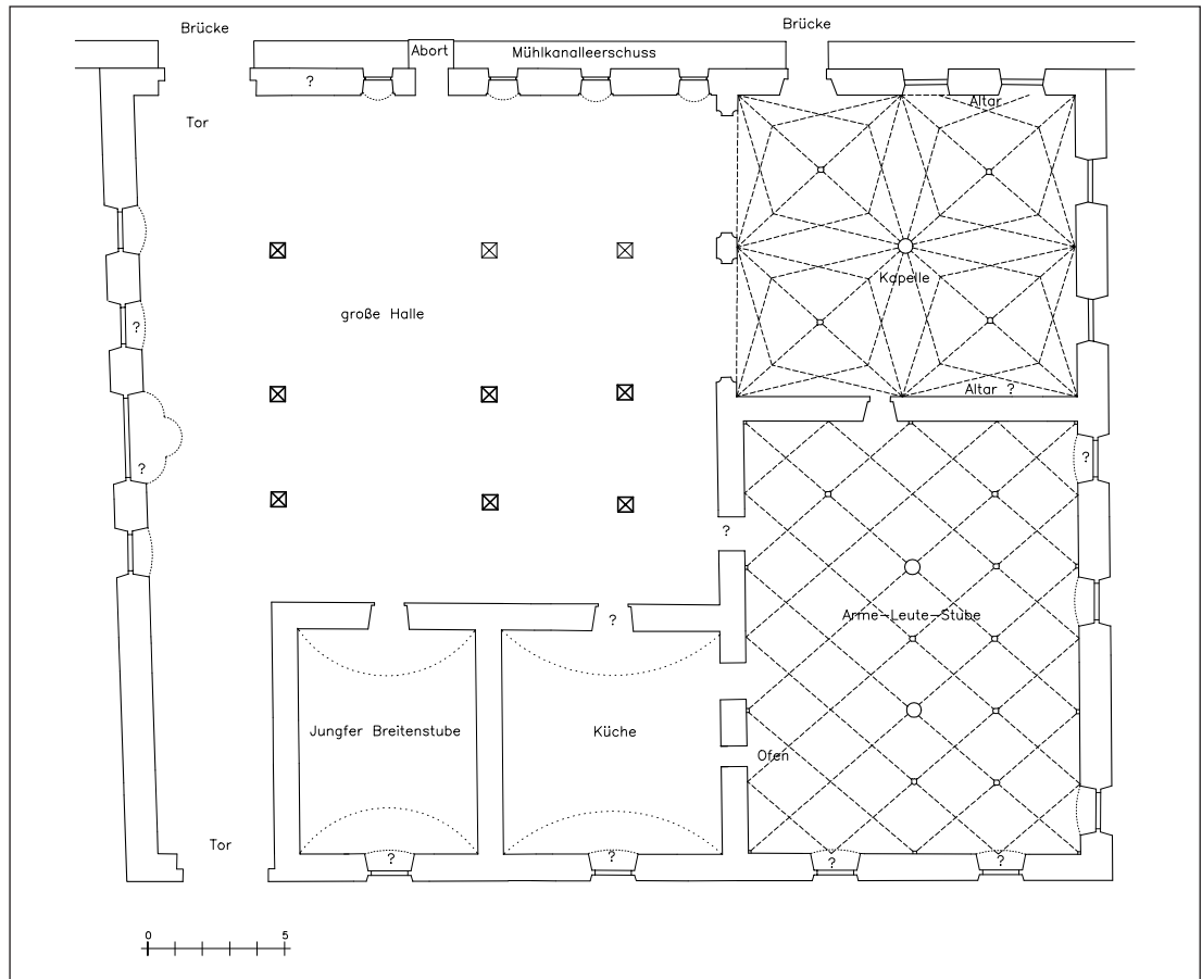
Abb. 1: Ravensburg, Heilig-Geist-Spital. Rekonstruktion um 1500, Erdgeschoss.
