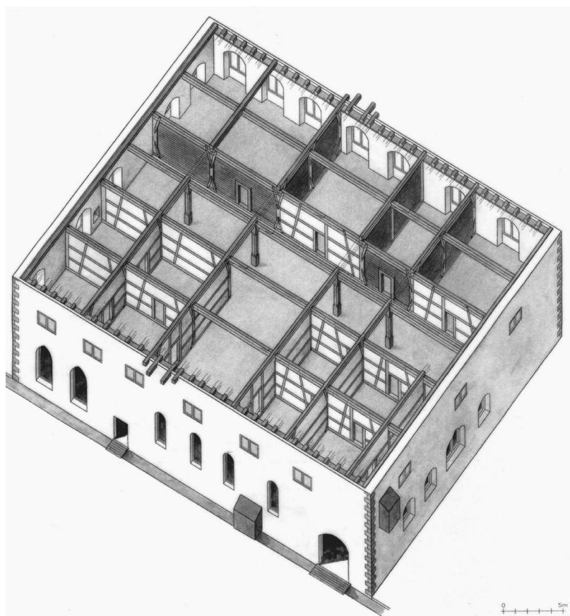
Abb. 4: Ravensburg, Heilig-Geist-Spital. Isometrische Rekonstruktion um 1500, 1. Obergeschoss.
