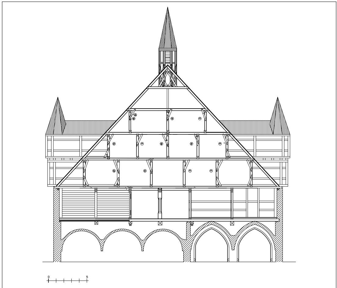
Abb. 5: Ravensburg, Heilig-Geist-Spital. Rekonstruktion um 1500, Querschnitt.
