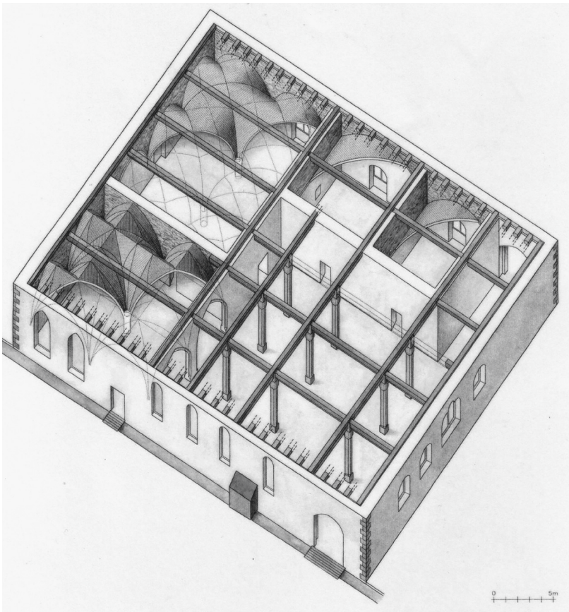
Abb. 2: Ravensburg, Heilig-Geist-Spital. Isometrische Rekonstruktion um 1500, Erdgeschoss.
