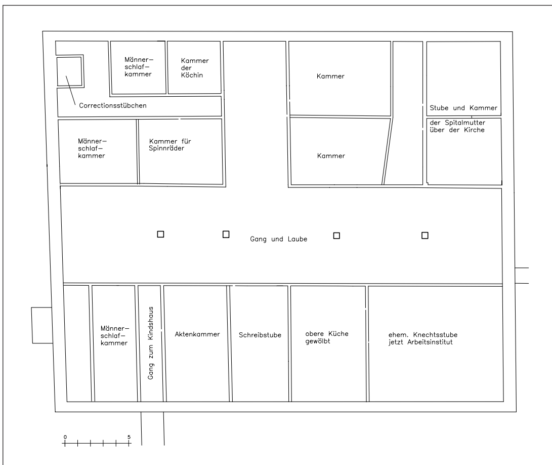
Abb. 8: Ravensburg, Heilig-Geist-Spital. Rekonstruktion um 1800, 1. Obergeschoss.
