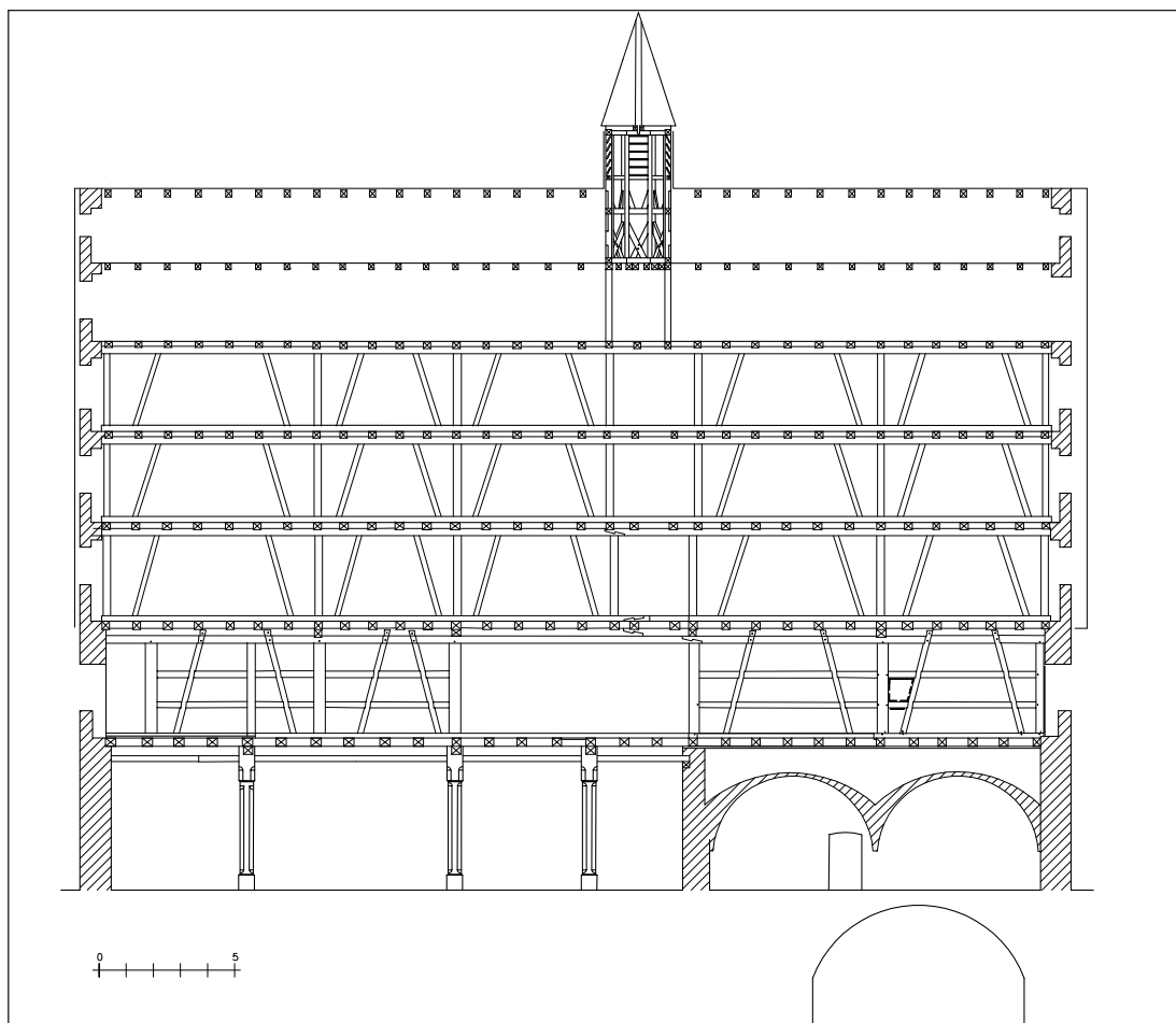
Abb. 6: Ravensburg, Heilig-Geist-Spital. Rekonstruktion um 1500, Längsschnitt.
