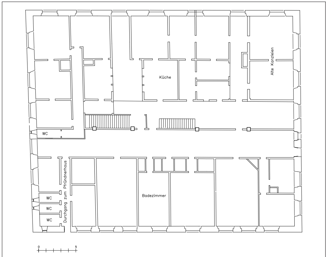
Abb. 9: Ravensburg, Heilig-Geist-Spital. Rekonstruktion von 1877, 1. Obergeschoss.
