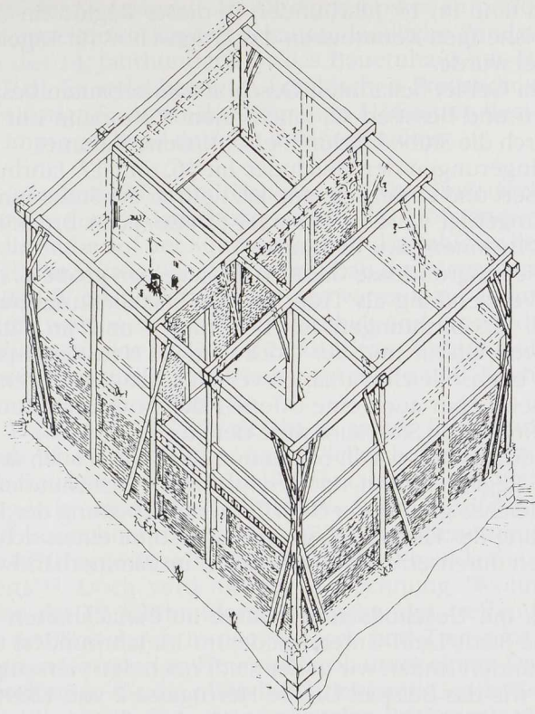
Abb. 7: Fichtenberg, Erlenhofer Str.10, isometrische Rekonstruktionsskizze des Geschößtänderbaues. Ansicht von Nordwesten. Die gestrichelten Bauteile sind Ergänzungen nach ersten Befunden, die durchgezogen dargestellten Bauteile sind vorhanden bzw. sicher zu rekonstruieren. Auch in diesem Haus finden wir nur eine Stube und die dahinter liegende Küche. Der westliche Hausteil wurde erst in späteren Zeiten mit Wänden aufgeteilt. Das Alter der Küchenabschlußwand zum Erschließungsbereich hin ließ sich noch nicht eindeutig klären, da das Anlegen von Oberflächenöffnungen hier nicht möglich waren. Das reine Dachgebälk wurde auf der Zeichnung fortgelassen
