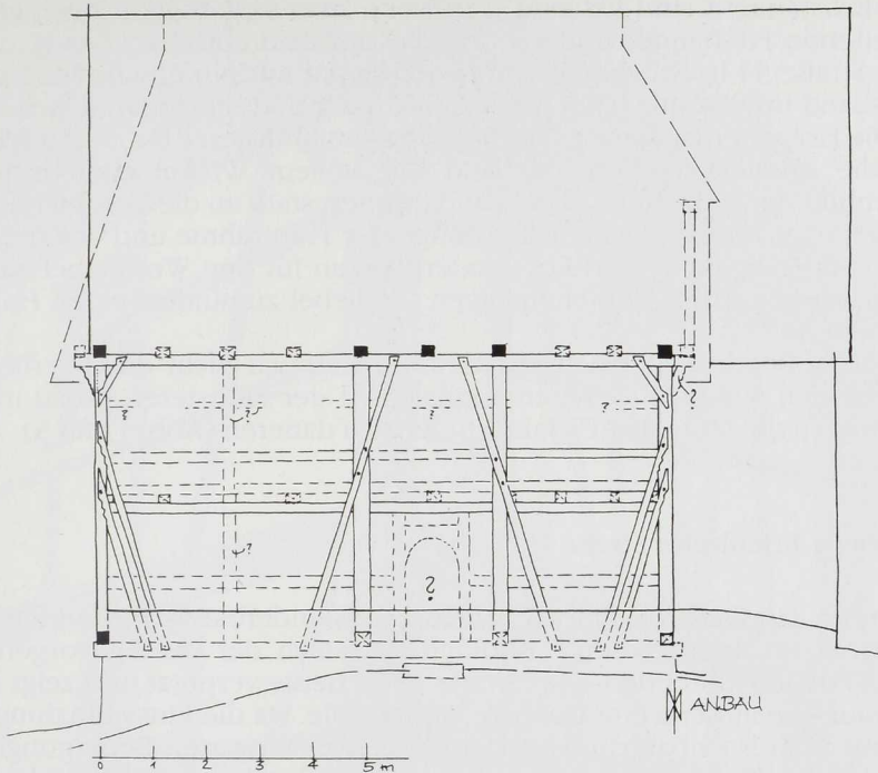
Abb. 4: Gaildorf-Münster, Spatzengasse/Ecke Brunnengasse, erster Rekonstruktionsversuch der Ostrauße nach äußerlichen Befunden. Auffallend sind die beiden Wandpfosten mit gegeneinander eingebauten Steigbändern über beide Geschosse. Die zum Teil noch vorhandenen Riegelfluchten im Obergeschoß sind ohne Nagelsicherung eingebaut.
