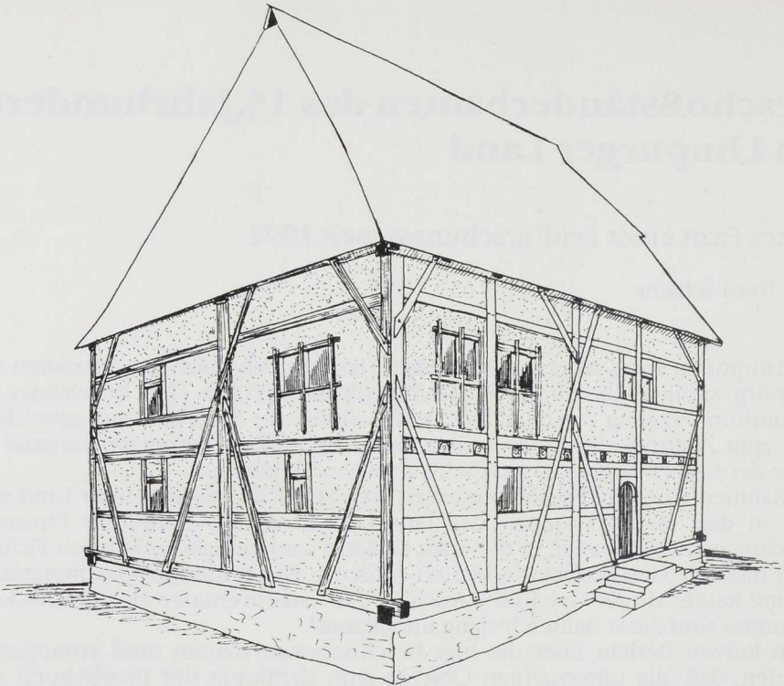
Abb. 1: Gaüldorf-Bröckingen, Aalener Straße 34, Rekonstruktionsversuch des Erstbaues, Ansicht von Südwesten. Ausgehend von den Anschlüssen der Ständer und Streben am südlichen Rähm und dem ablesbaren Bestand an der Westseite ergab sich dieses Rekonstruktionsbild. Die Stube und die Küche liegen bei diesem Haus auf der Westhälfte des Grundrisses. Die Fensteranlagen der Stube und die Haustürform sind frei ergänzt.
