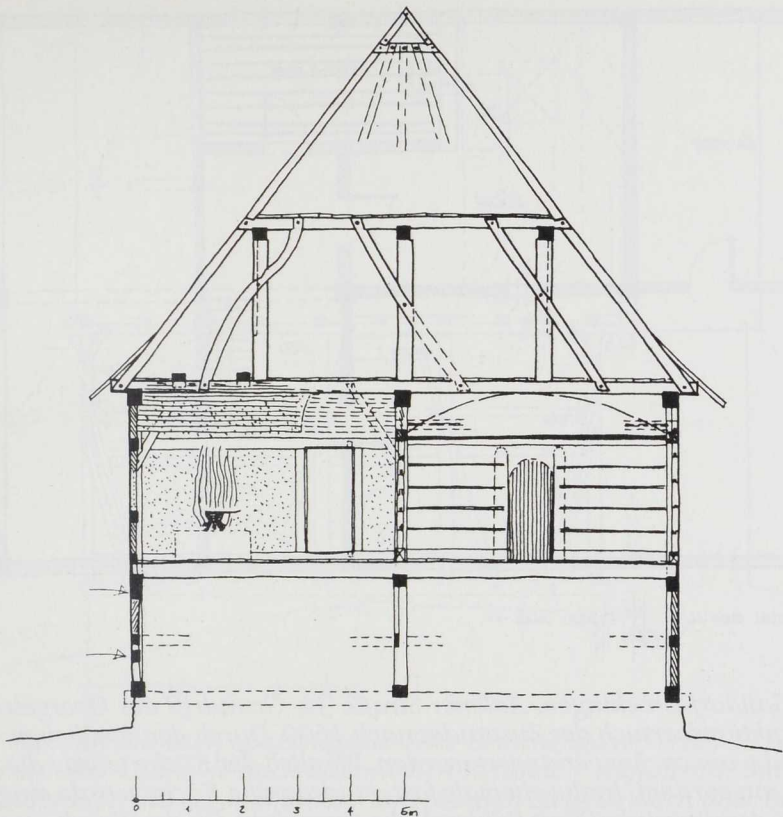
Abb. 2: Gaildorf-Bröckingen, Aalener Straße 34, Schnitt hinter dem Westgiebel, Blickrichtung nach Osten. Noch heute steht am Platz der einstmaligen Feuerstelle ein holzbefuener Sparherd. Die ehemalige Hurt wurde in der Zeichnung zur Stube hin ergänzt; ebenso das Türgewände und die rundbogige Stubentüre in der nachgewiesenen Bohlenwand. Ob die Stubendecke tatsächlich gewölbt war, wie erste Beobachtungen ergaben, kann erst nach vollständiger Einsichtnahme in den Deckenhohlraum geklärt werden.
