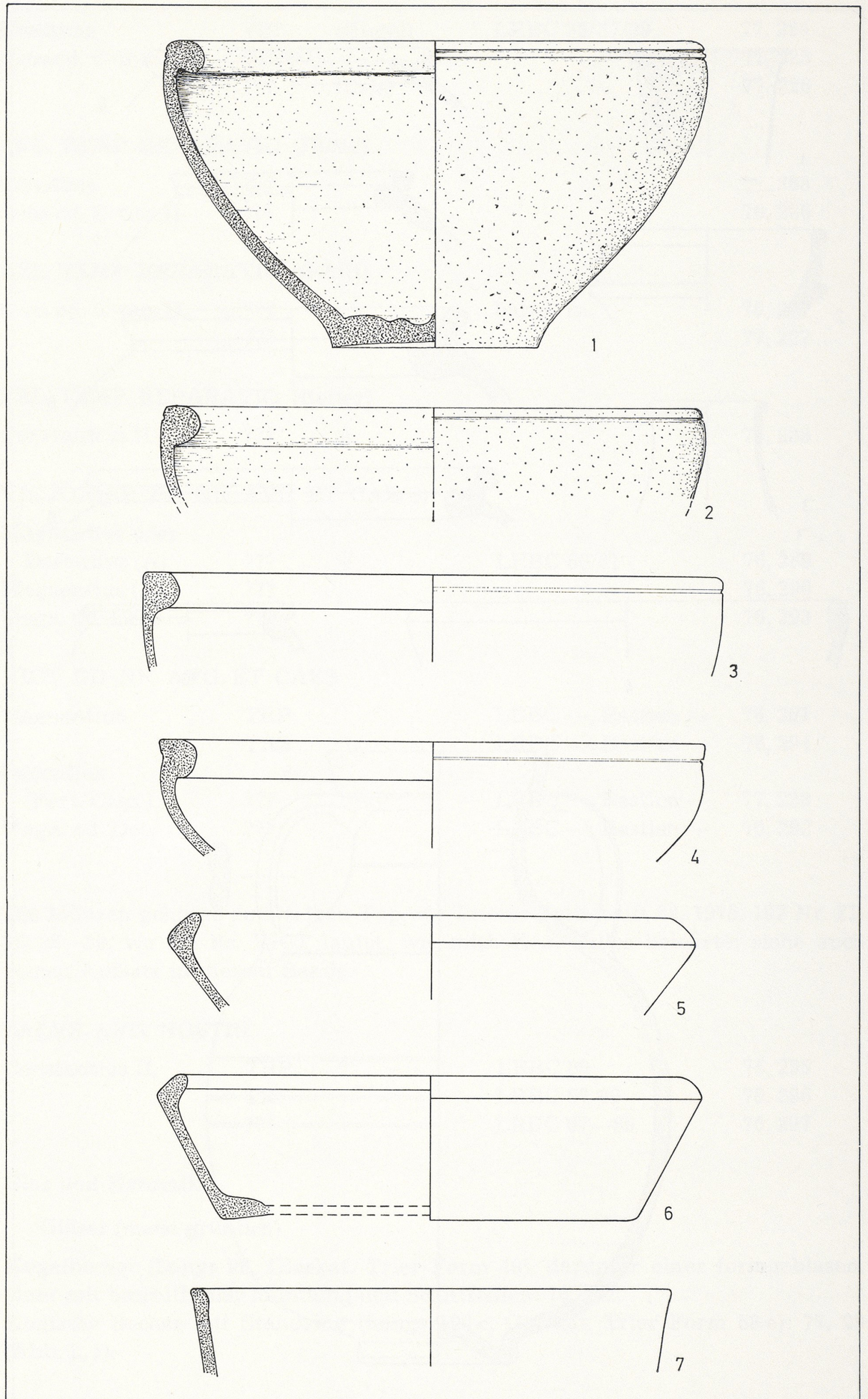
Abb. 2 Bengel, Keramik. 1:4
