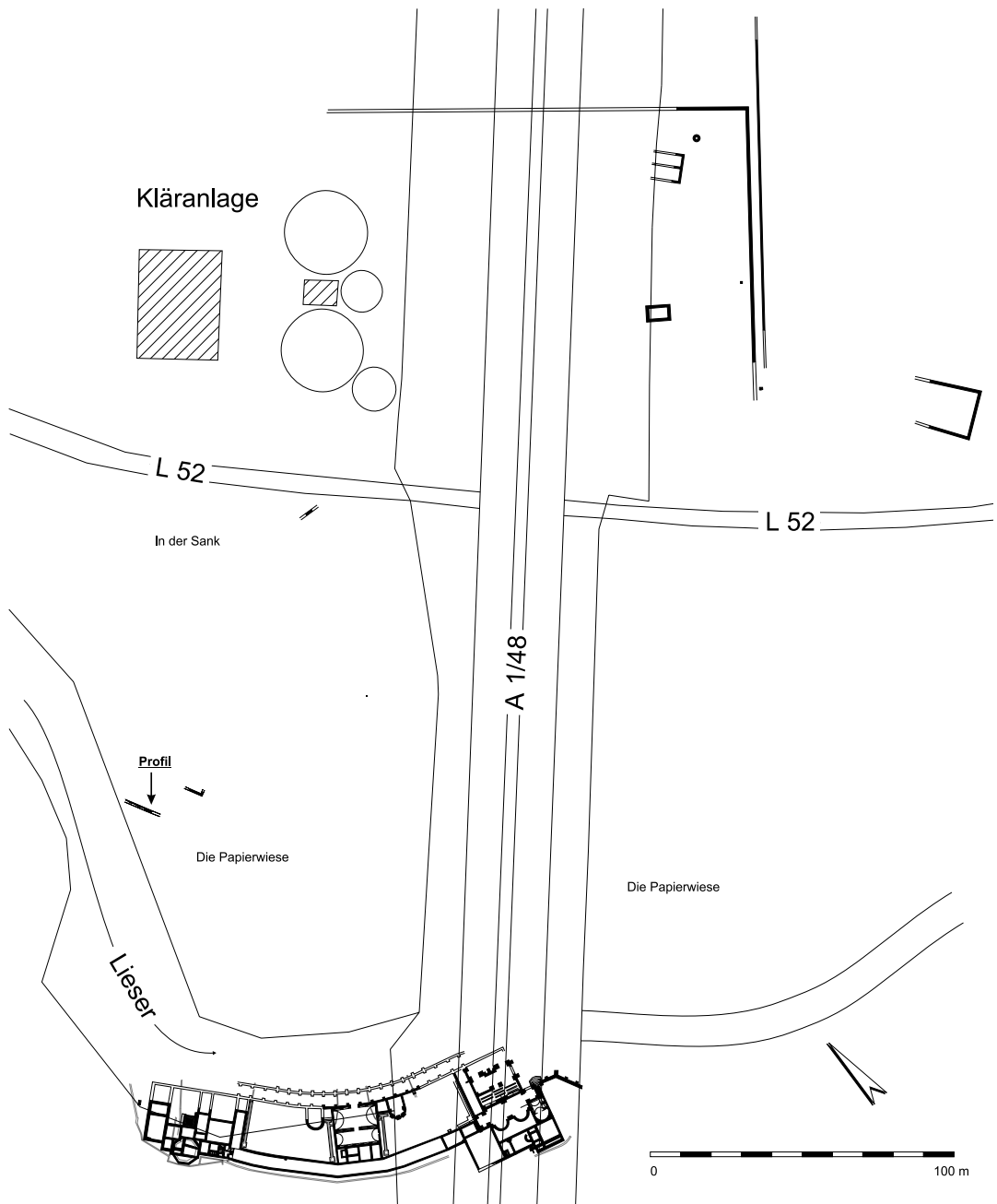
Abb. 13 Wittlich. Grundriß der römischen Villa mit ihrem Wirtschaftsbereich und den in der „Papierwiese“ neu nachgewiesenen Mauerzügen. (Zeichnung: O. Haffner).
