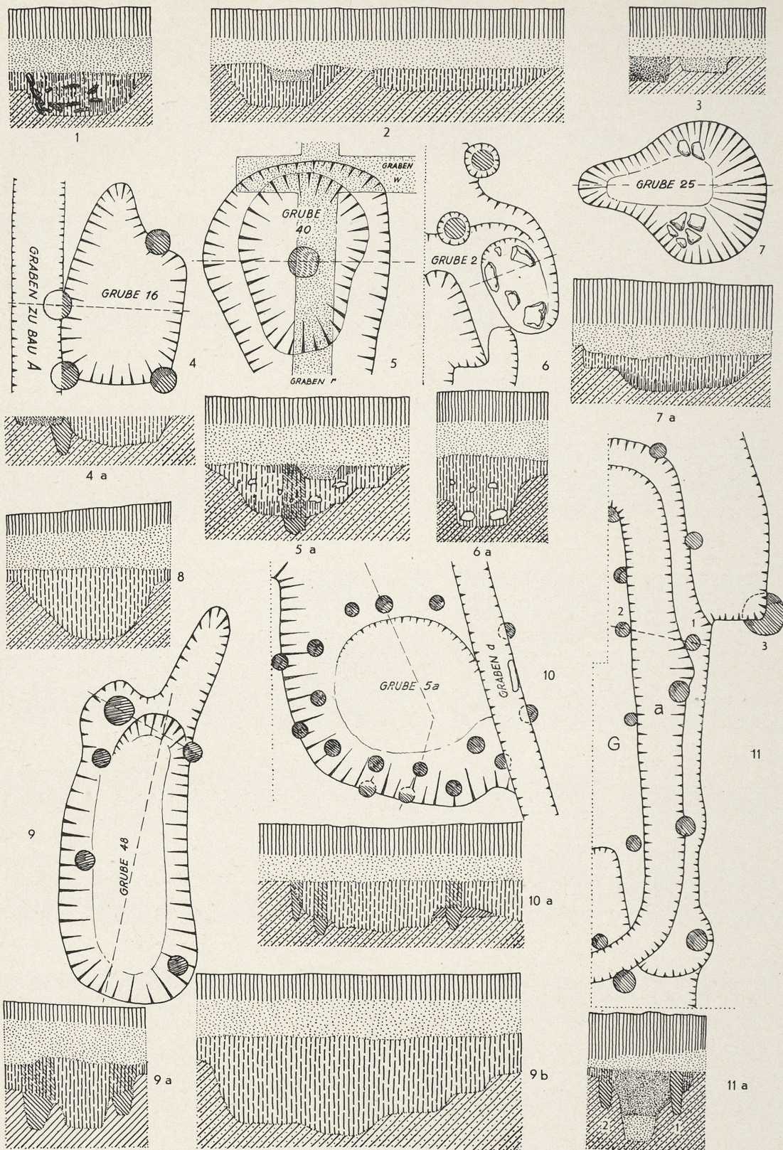
Bernkastel-Kues. Teilpläne und Schnitte (s. Legende S. 53 f.). M 1:50 (Nr. 10 M 1:40)
