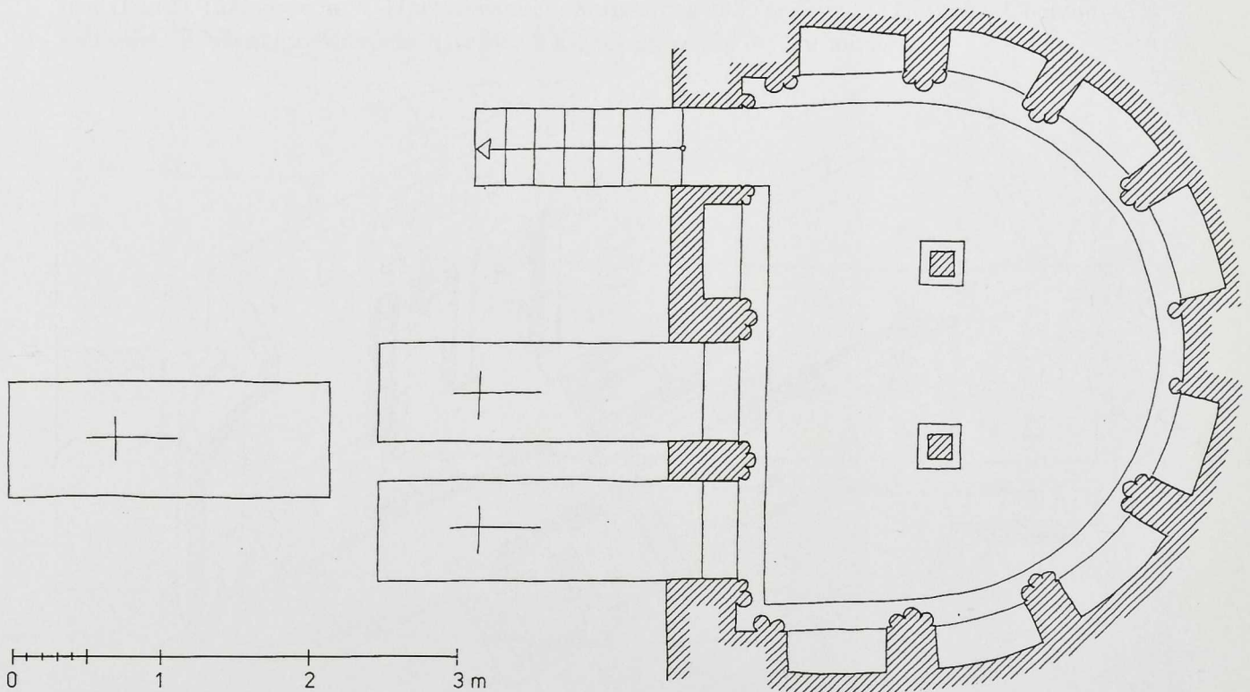
Abb. 11 Quedlinburg, Stiftskirche St. Servatii, »Confessio« und Königsgräber, Rekonstruktionsversuch des Grundrisses (1:60). An die Westwand schloß im Norden (oben) das Zugangstrepptchen, in der Mitte der Königssarg an. Südlich von ihm befindet sich noch heute der Sarg der Königin (unten) und westlich von beiden der der Äbtissin Mathilde.
