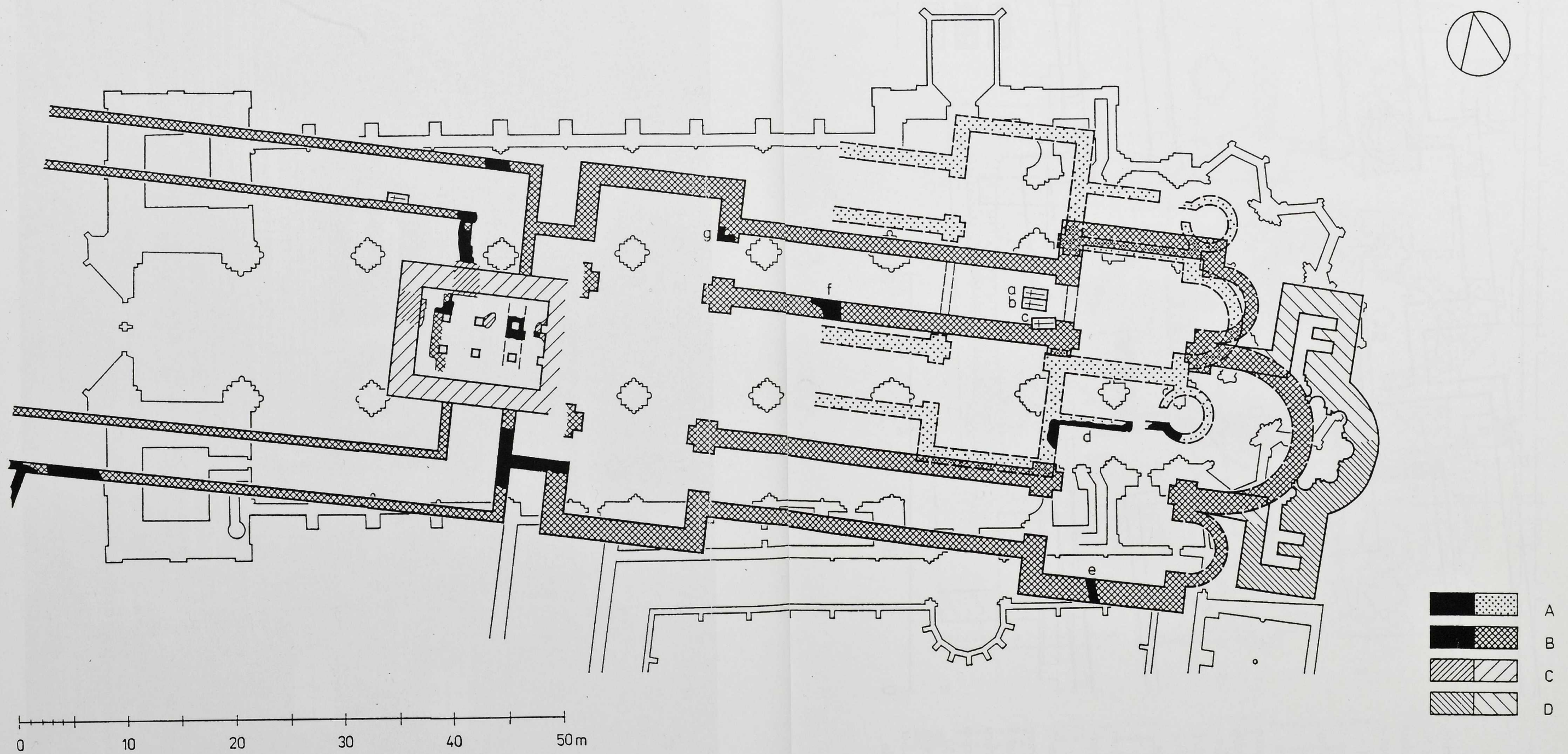
Abb. 28 Magdeburg, Dom, Grundriß (1:500) der Moritz-Klosterkirche und des ottonischen Doms, Rekonstruktionsversuch
