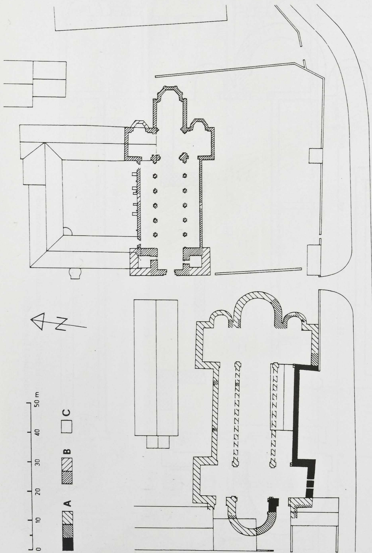
Abb. 22 Memleben, Lageplan (1:1000) des Ruinengeländes A Ottonische Kirche: aufgehend/ergraben/ergänzt, B Kirche des 13. Jahrhunderts: aufgehend/ergänzt, C Gebäude des Gutes
