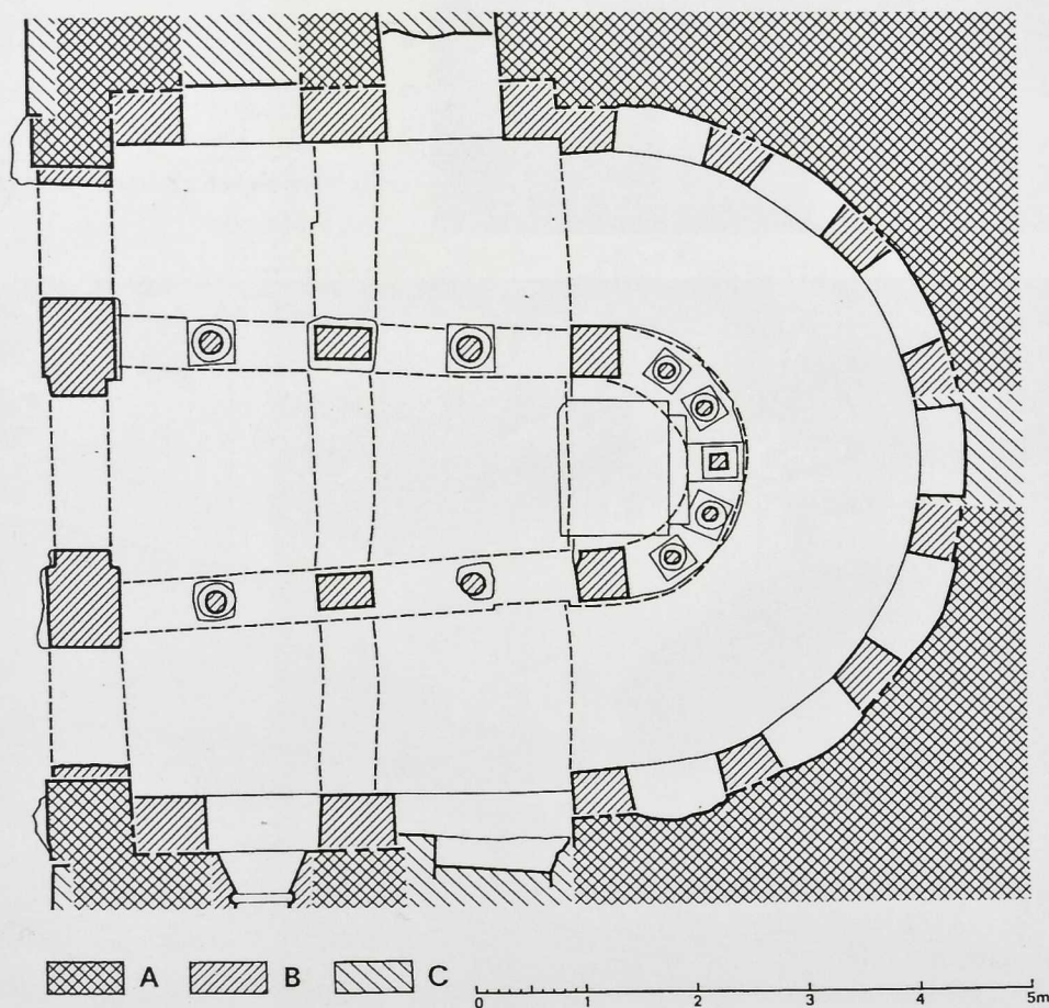
Abb. 19 Quedlinburg, St. Wiperti, Grundriß (1: 100) der Krypta mit Bauzeiten
