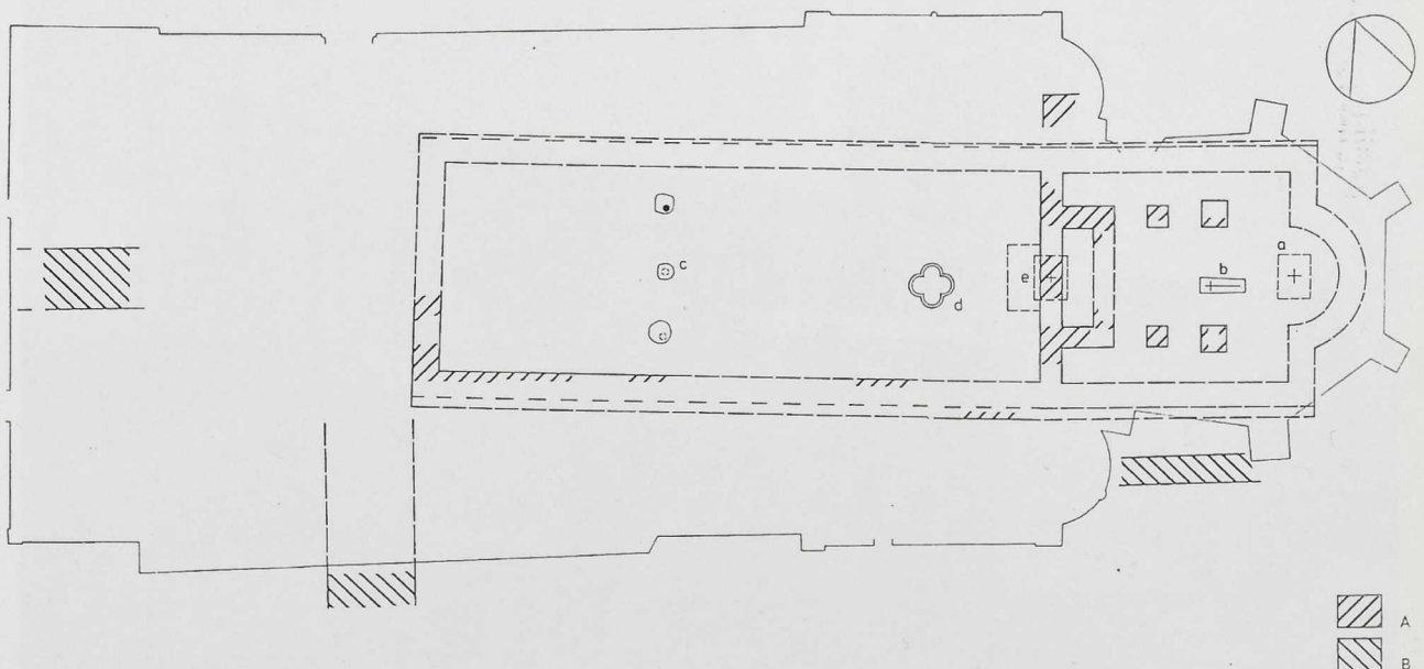
Abb. 7 Quedlinburg, Stiftskirche St. Servatii, Grundriß (1:500) der Burgkapelle König Heinrichs I. (Bau 1), Rekonstruktionsversuch A Nachgewiesenes Mauerwerk der Kapelle, B Neben ihr nachgewiesene Mauerreste, a Petrus-Altar, b Grab König Heinrichs I., c Pfostenlöcher, d Taufbecken, e Möglicher Standort des Hauptaltars
