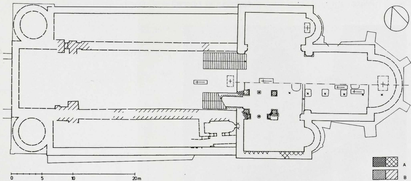
Abb. 18 Quedlinburg, Stiftskirche St. Servatii, Grundriß (1:500) der 1021 geweihten Kirche (Bau 3), unten in Höhe der Krypta, oben in Höhe des Chors, Rekonstruktionsversuch
