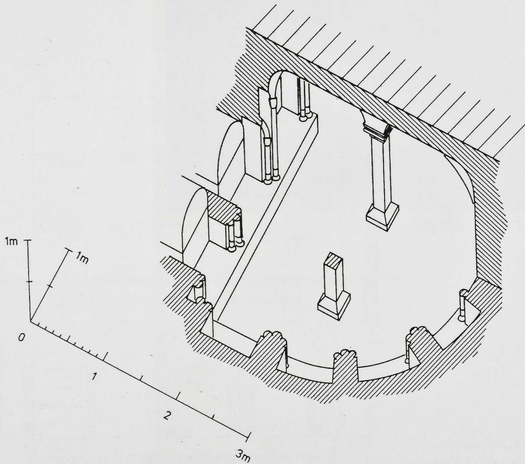
Abb. 13 Quedlinburg, Stiftskirche St. Servatii, »Confessio«, isometrischer Rekonstruktionsversuch
