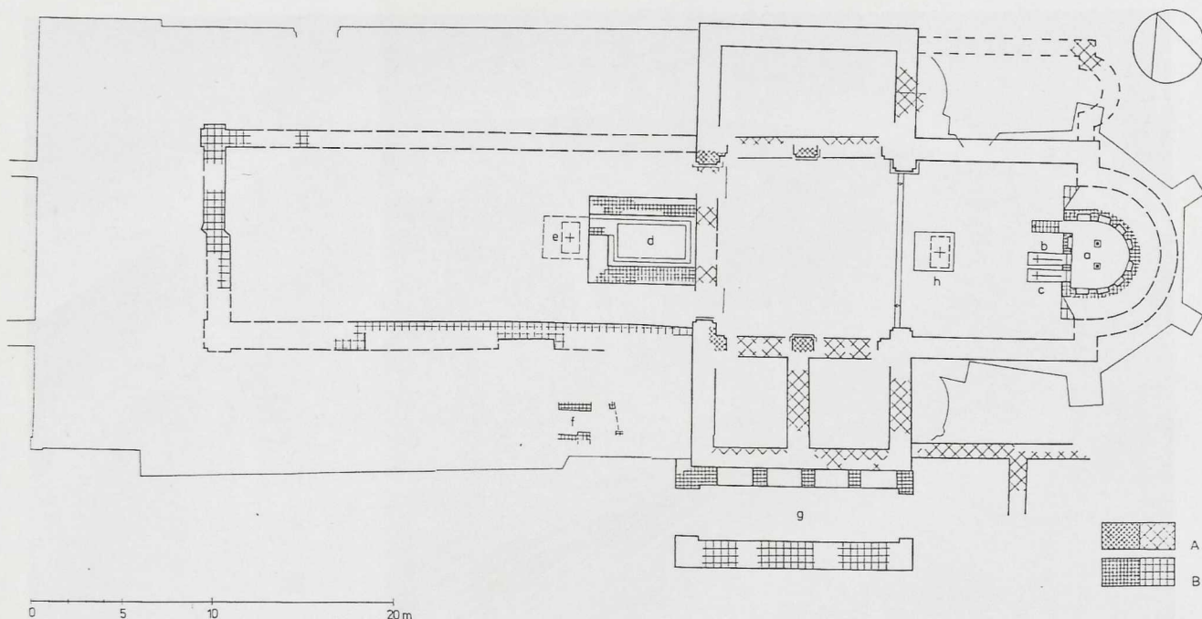
Abb. 8 Quedlinburg, Stiftskirche St. Servatii, Grundriß (1:500) der Kirche der Königin Mathilde (Bau 2), Rekonstruktionsversuch
