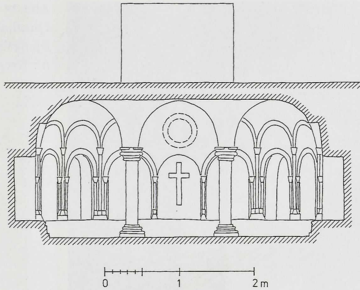
Abb. 12 Quedlinburg, Stiftskirche St. Servatii, Schnitt (1:60) nach Osten durch die »Confessio«, Rekonstruktionsversuch
