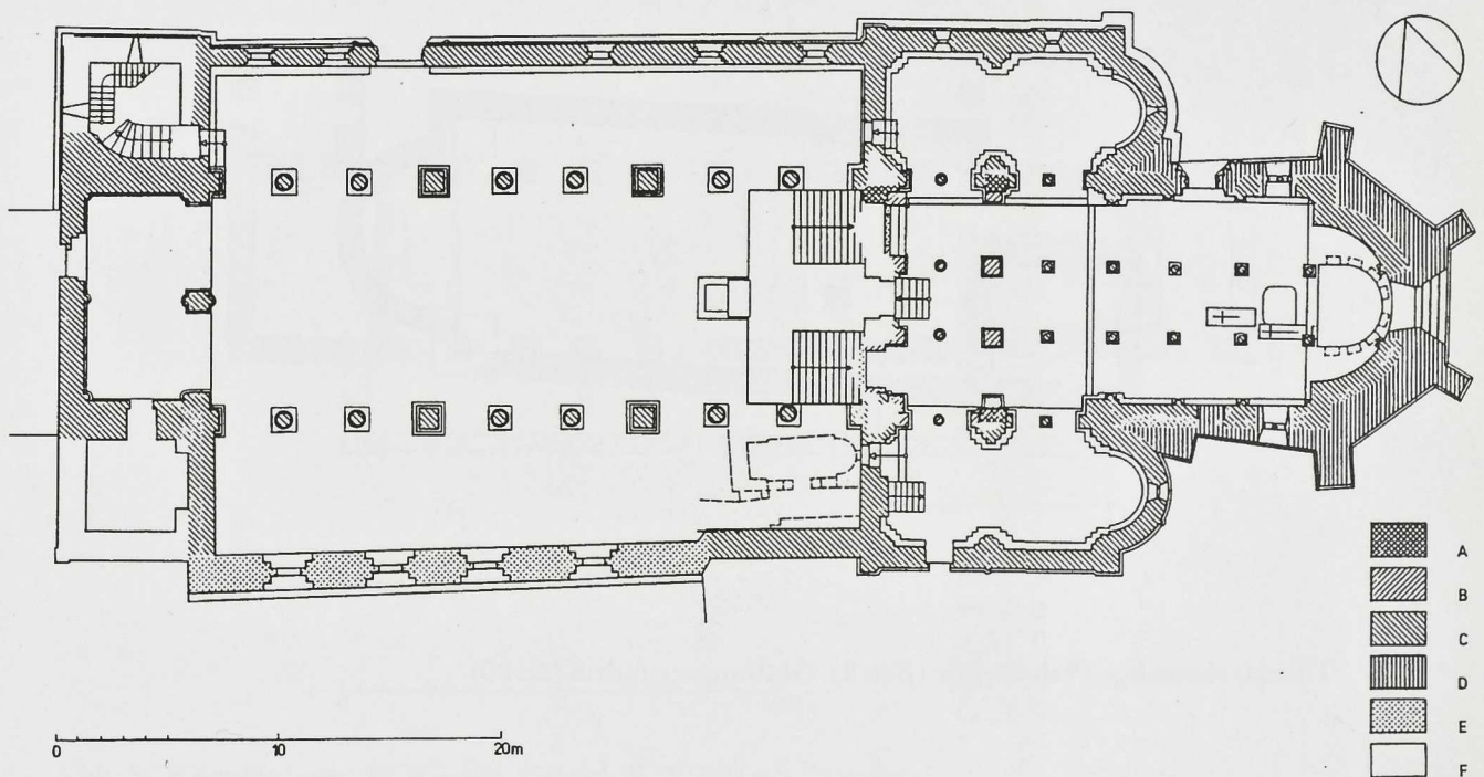
Abb. 6 Quedlinburg, Stiftskirche St. Servatii, Grundriß (1:500) mit Bauzeiten A Stiftskirche der Königin Mathilde (Bau 2), nach 936, B Stiftskirche der Äbtissinnen Mathilde und Adelheid (Bau 3), 1021 geweiht, C Hochromanische Stiftskirche, 1129 geweiht, D Gotischer Chor, um 1320 vollendet, E Nachmittelalterliche Bauteile, F Ergänzungen des 19. Jahrhunderts
