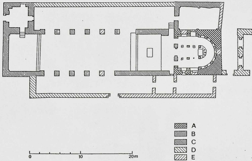
Abb. 2 Quedlinburg, St. Wiperti, Grundriß (1:500) mit Bauzeiten
