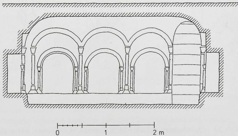
Abb. 15 Quedlinburg, Stiftskirche St. Servatii, Schnitt (1:60) nach Westen durch die »Confessio«, Rekonstruktionsversuch
