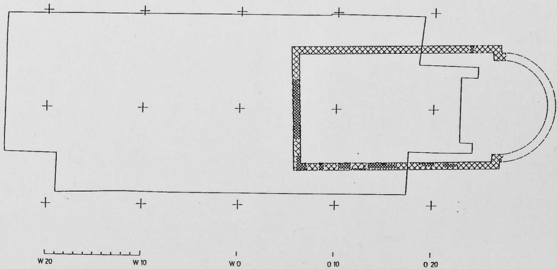
Abb. 3 Quedlinburg, St. Wiperti, Grundriß (1:500) der Kapelle Heinrichs I. (Bau 1), Rekonstruktionsversuch
